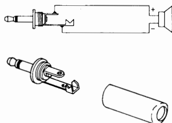
外部スピーカープラグの接続
