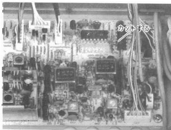
KEYER UNIT B取付前
