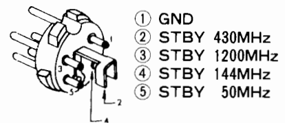
STBYプラグの接続
