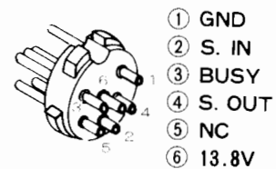
CATプラグの接続
