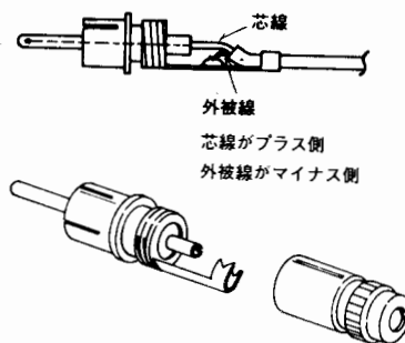
PTTプラグの接続
