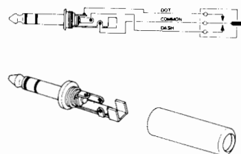
KEYプラグの接続
