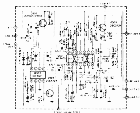
第8図 Tone Squelch回路図
