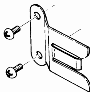
第2図 マイクハンガの取り付け方
