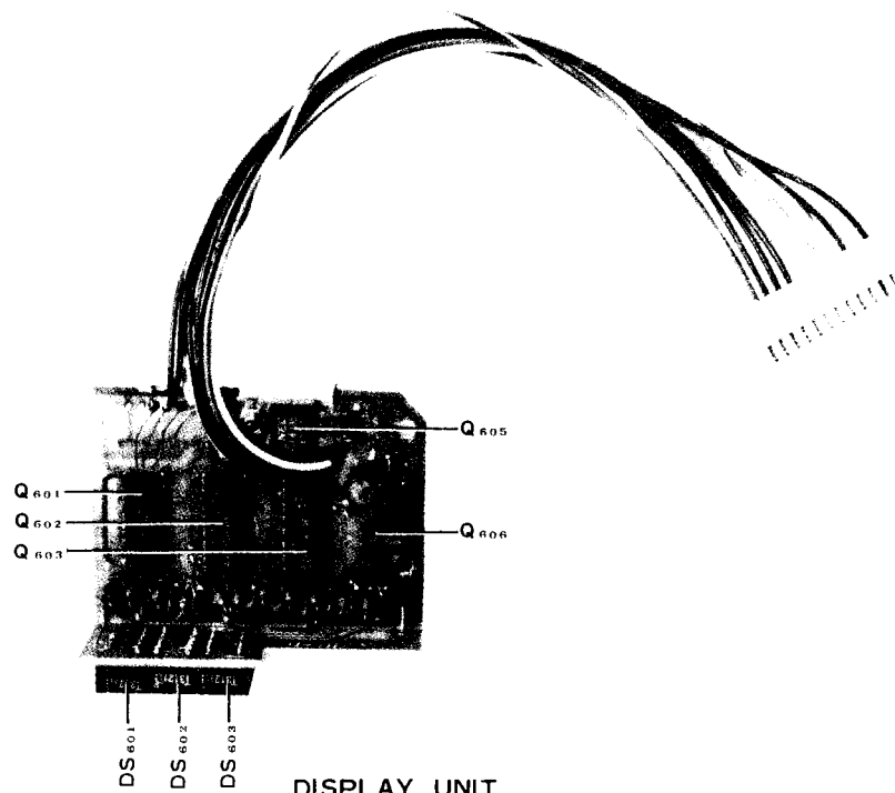
DISPLAY UNIT
