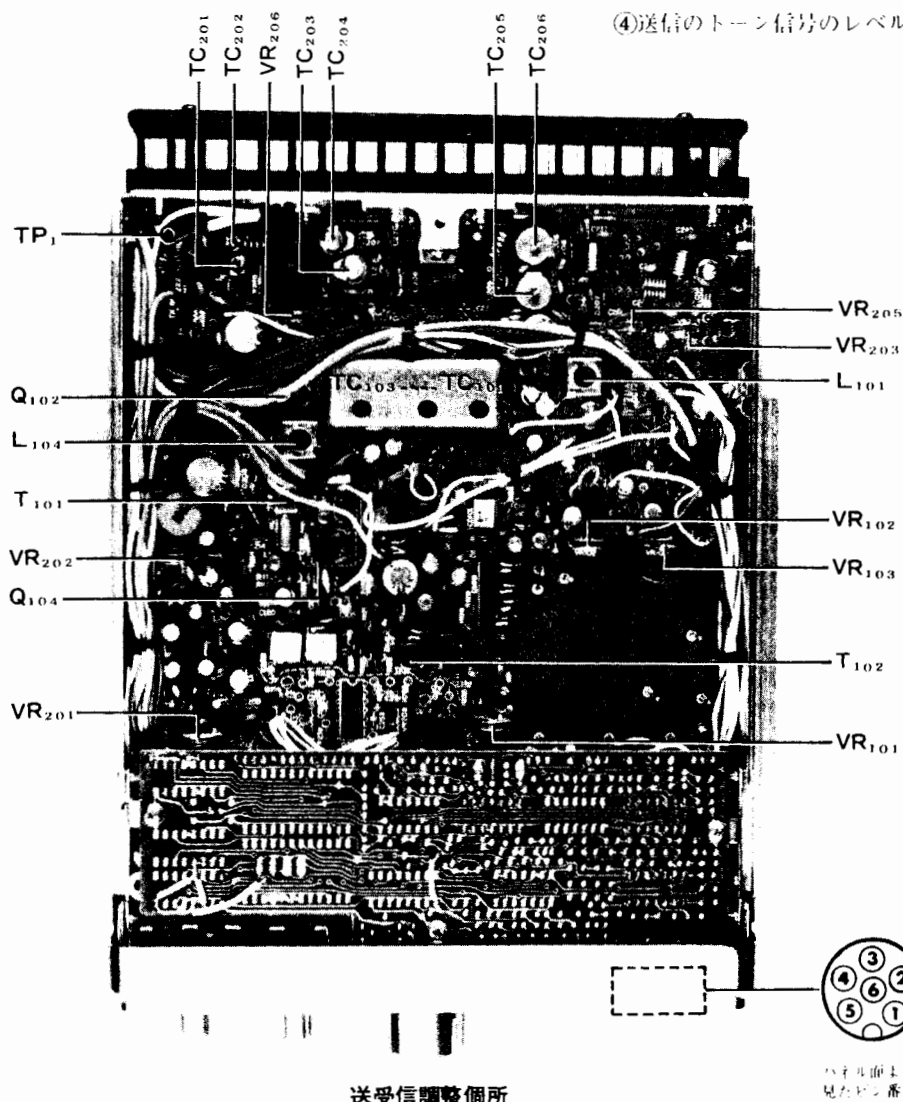
送受信調整箇所
