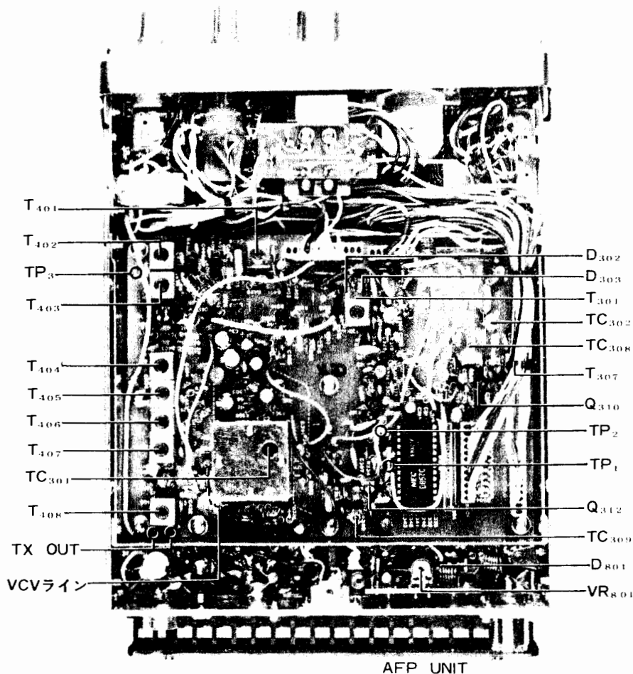
PLL 部調整箇所
