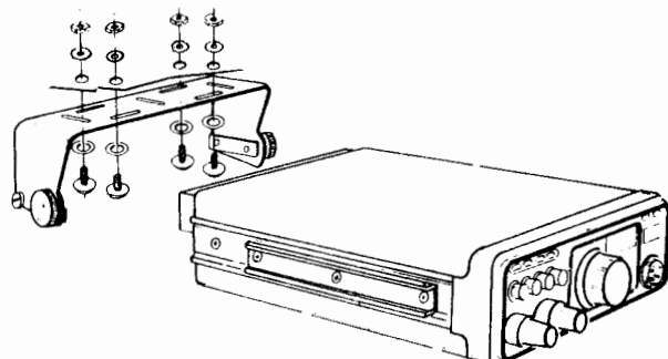
第3図 セットの取り付け方
