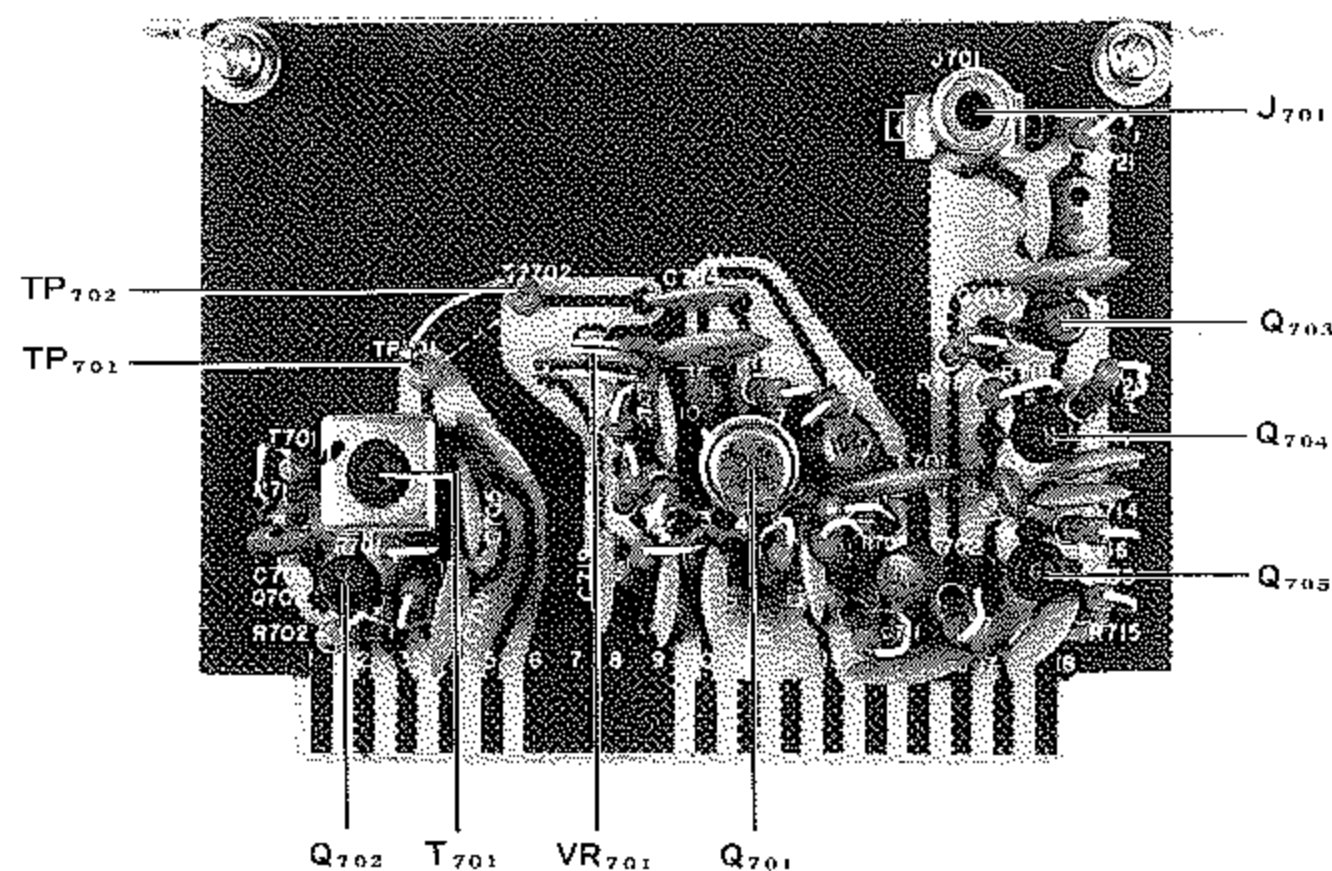
PREMIX UNIT (PB-1439)
