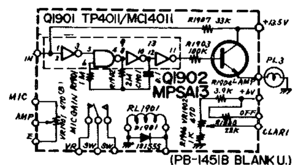
第20図 BLANKING UNIT (PB-1451B)
