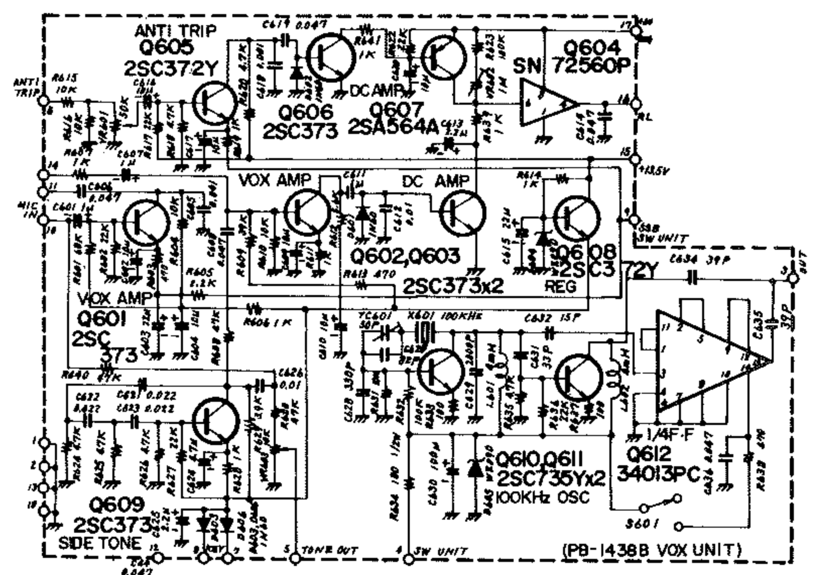
第21図 VOX UNIT (PB-1438B)
