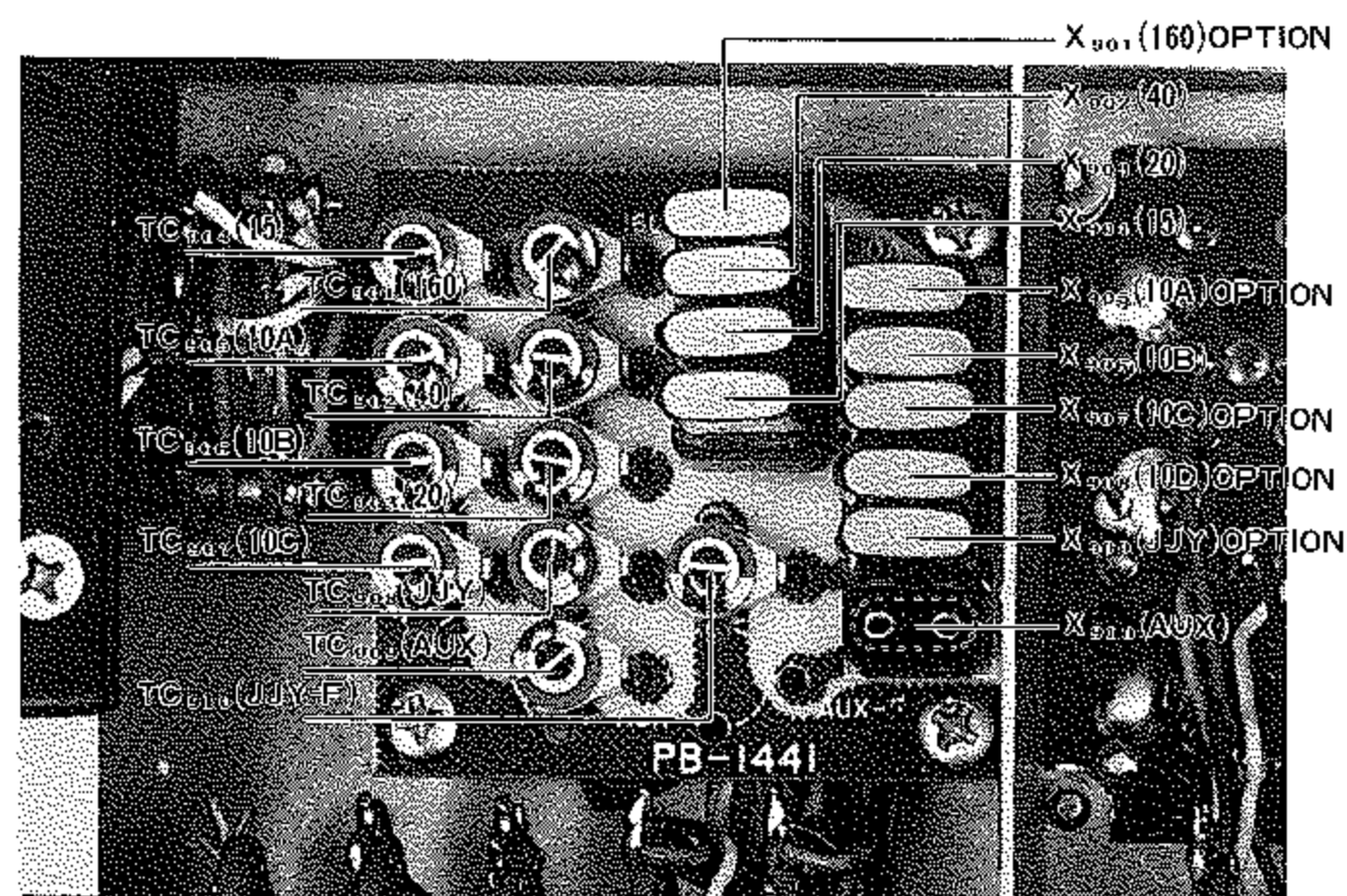
CRYSTAL UNIT (PB-1441)
