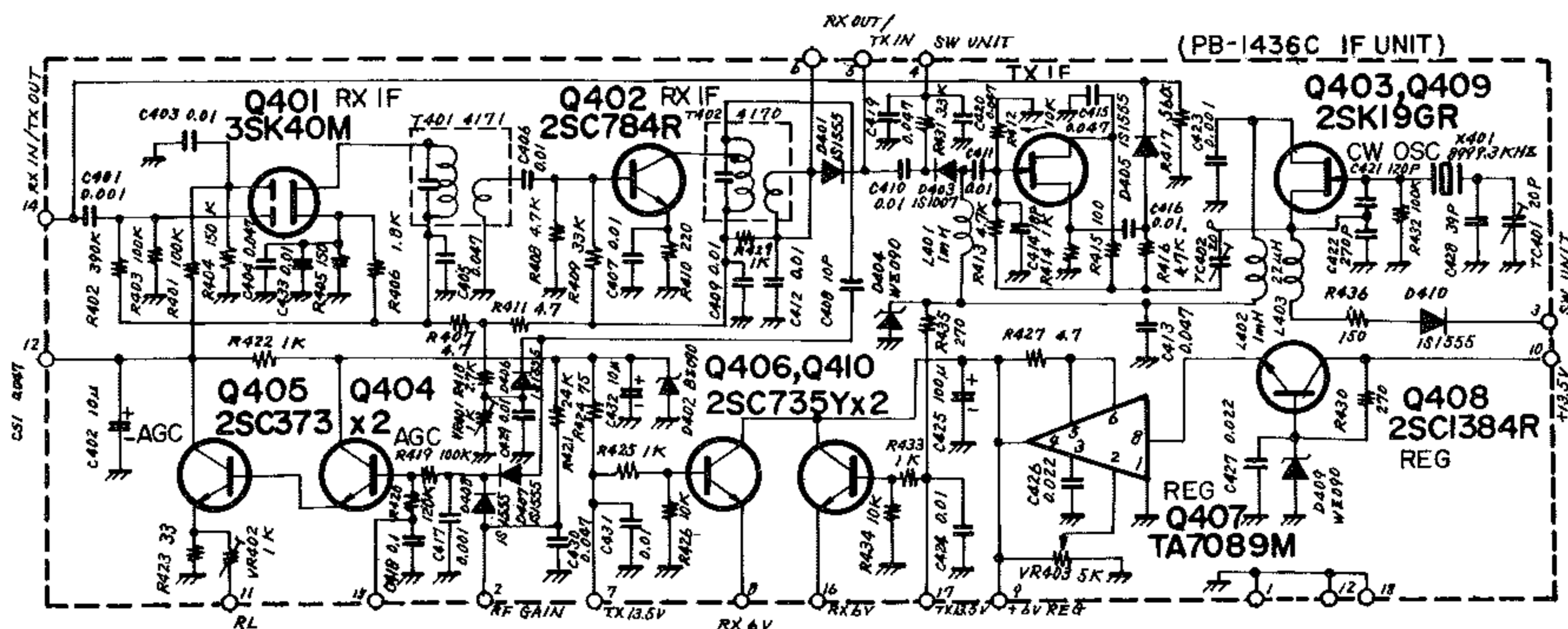
第12図 IF UNIT (PB-1436C)
