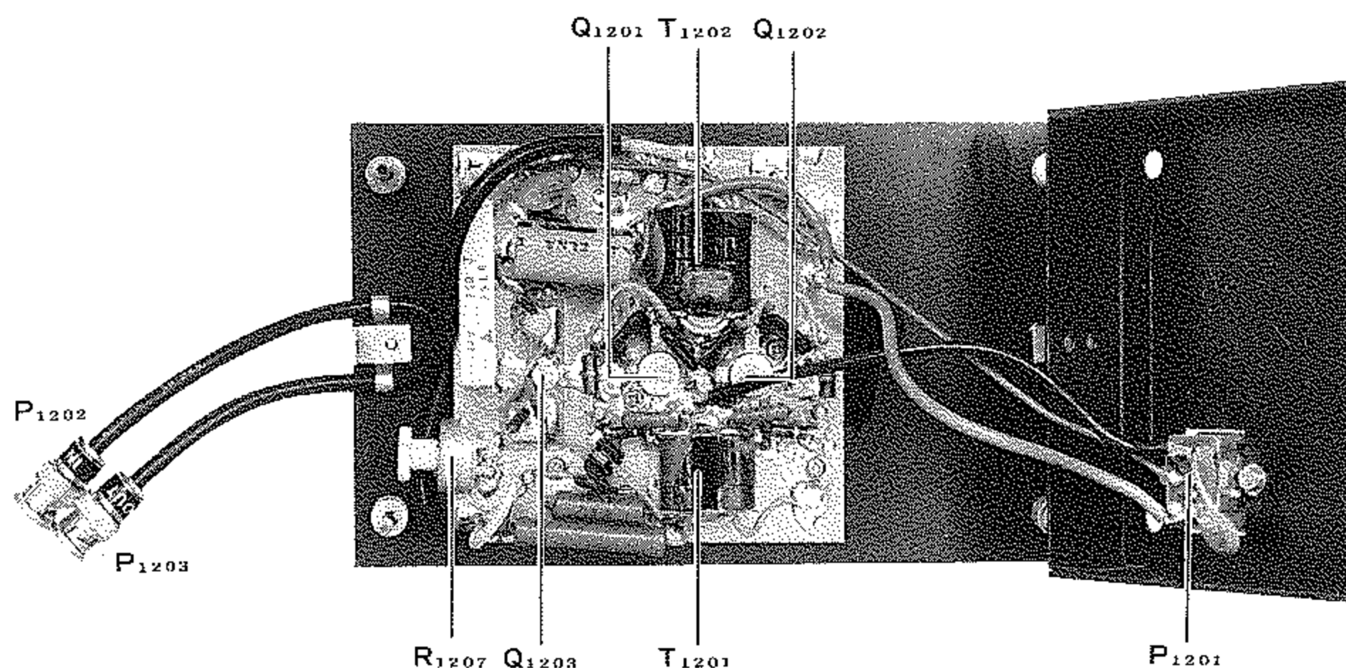
BOOSTER UNIT (PB-1444)
