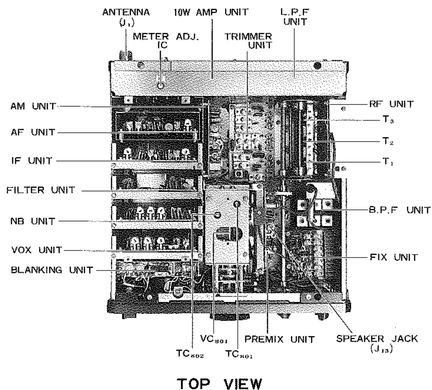
FT-301S 内部写真
