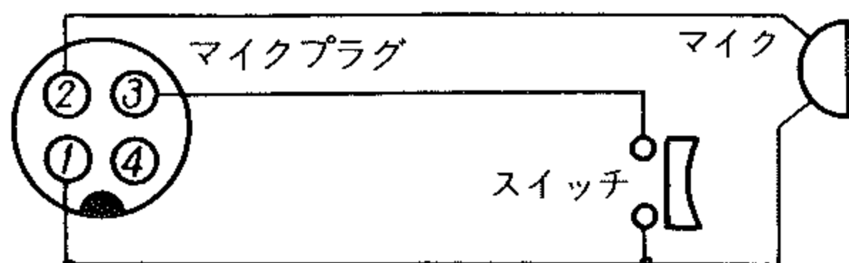
第1図 マイクの接続
