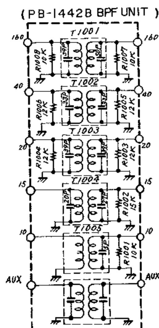
第26図 BPF UNIT (PB-1442B)
