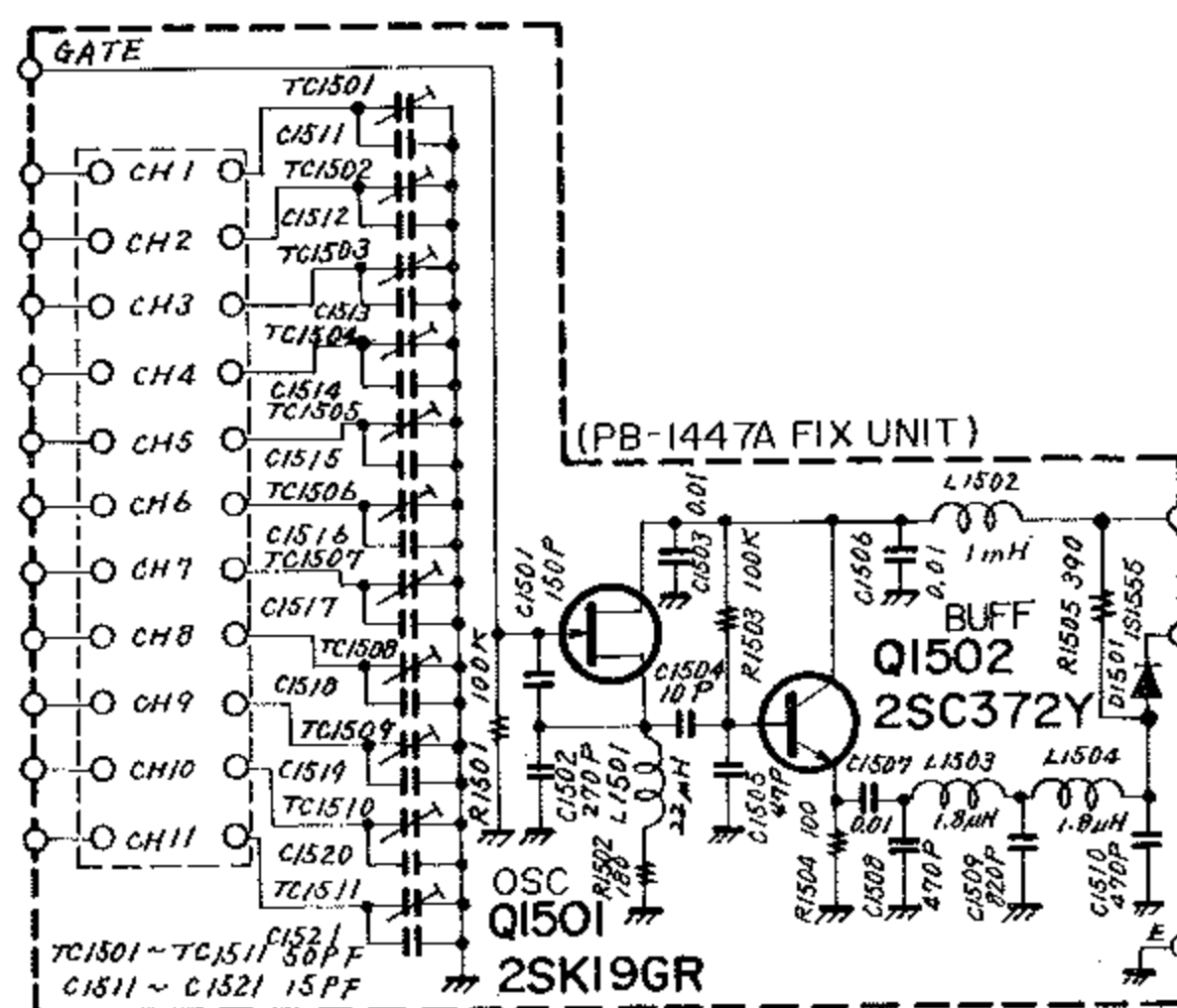
第23図 FIX UNIT (PB-1447A)
