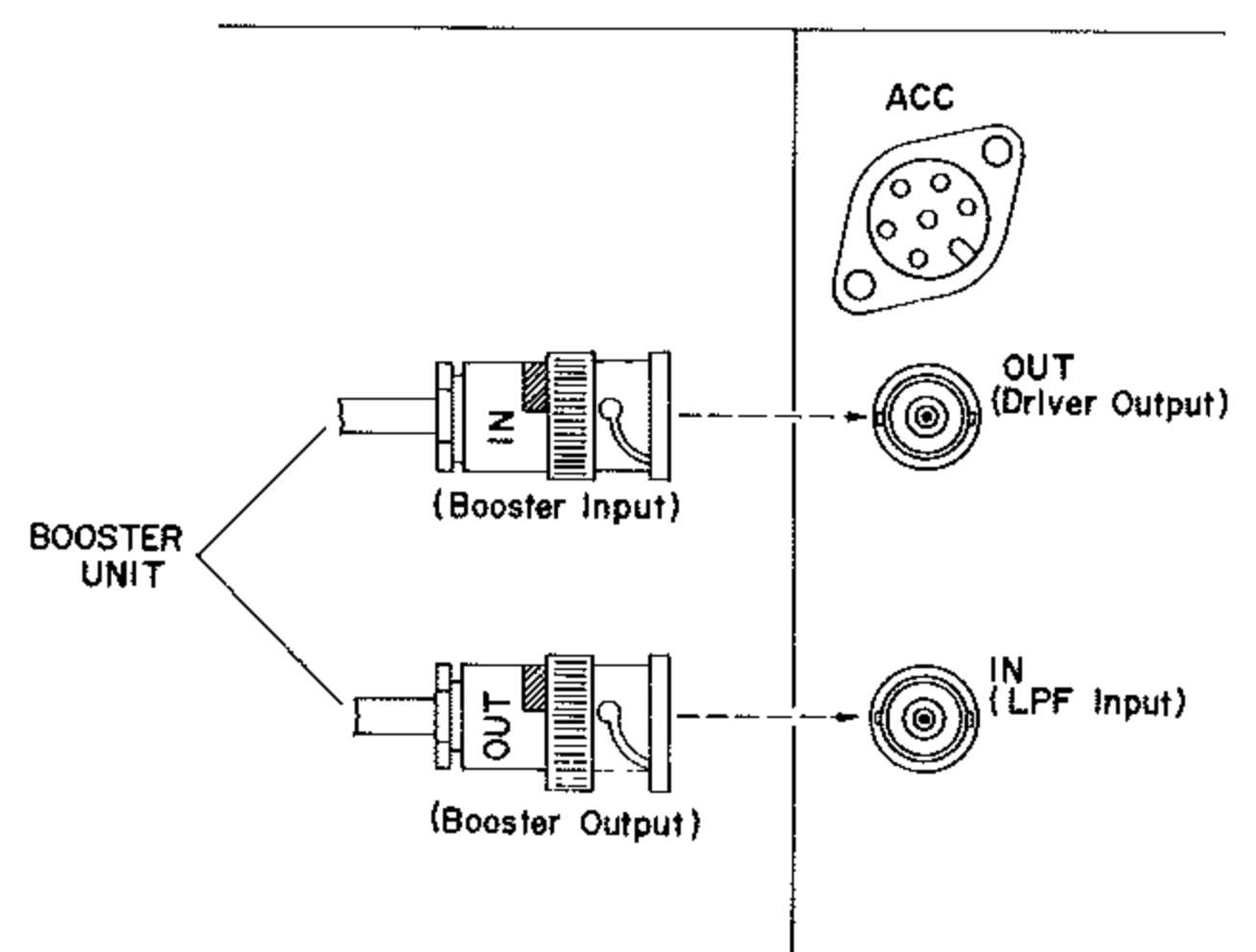
第5図 ブースタコネクタの接続
