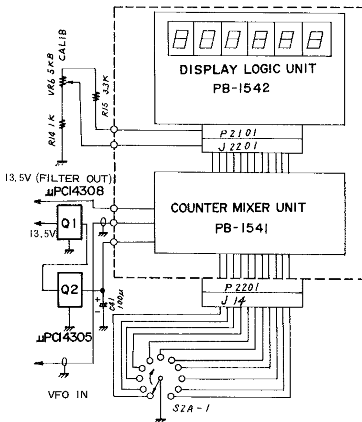
第28図 FT-301SDのFT-301S回路図に追加の部分
