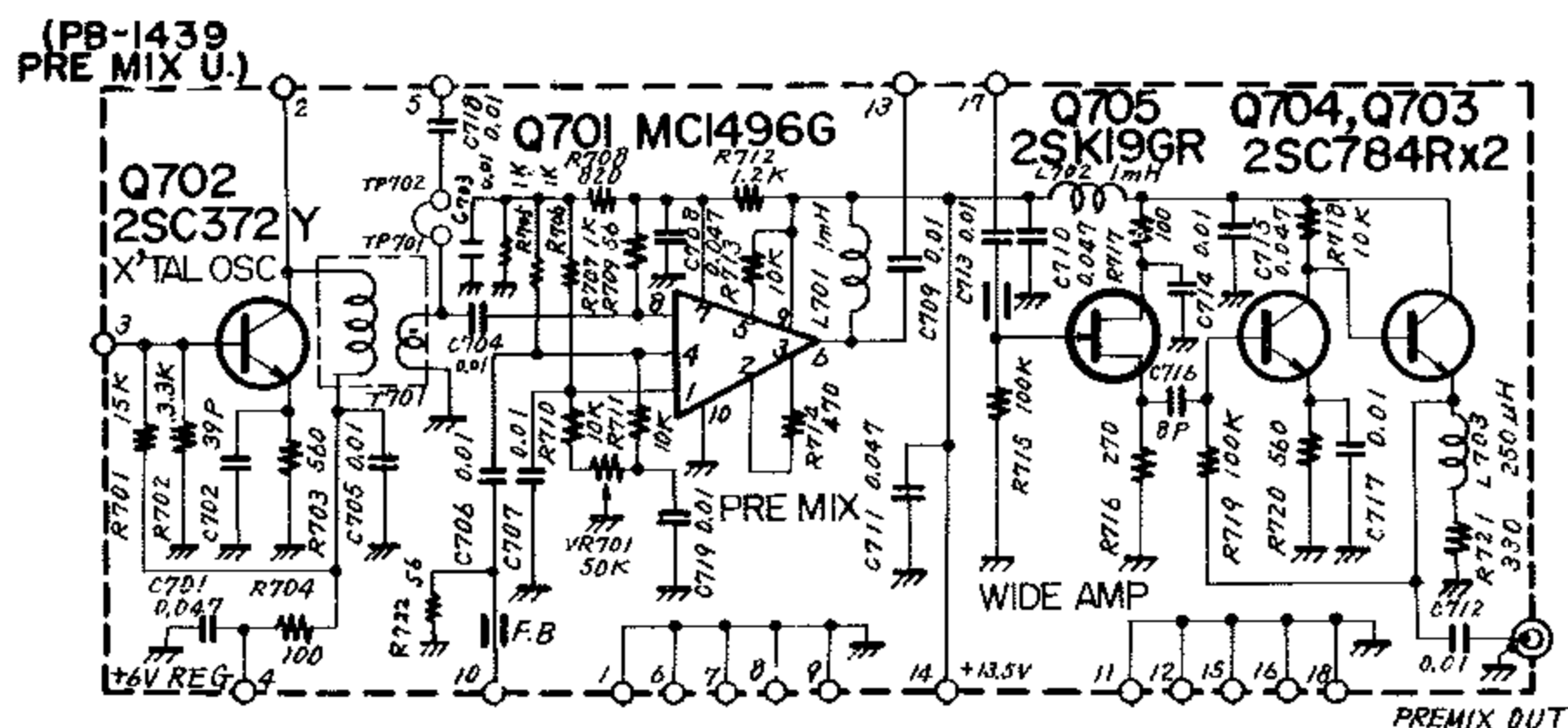
第24図 PREMIX UNIT (PB-1439)
