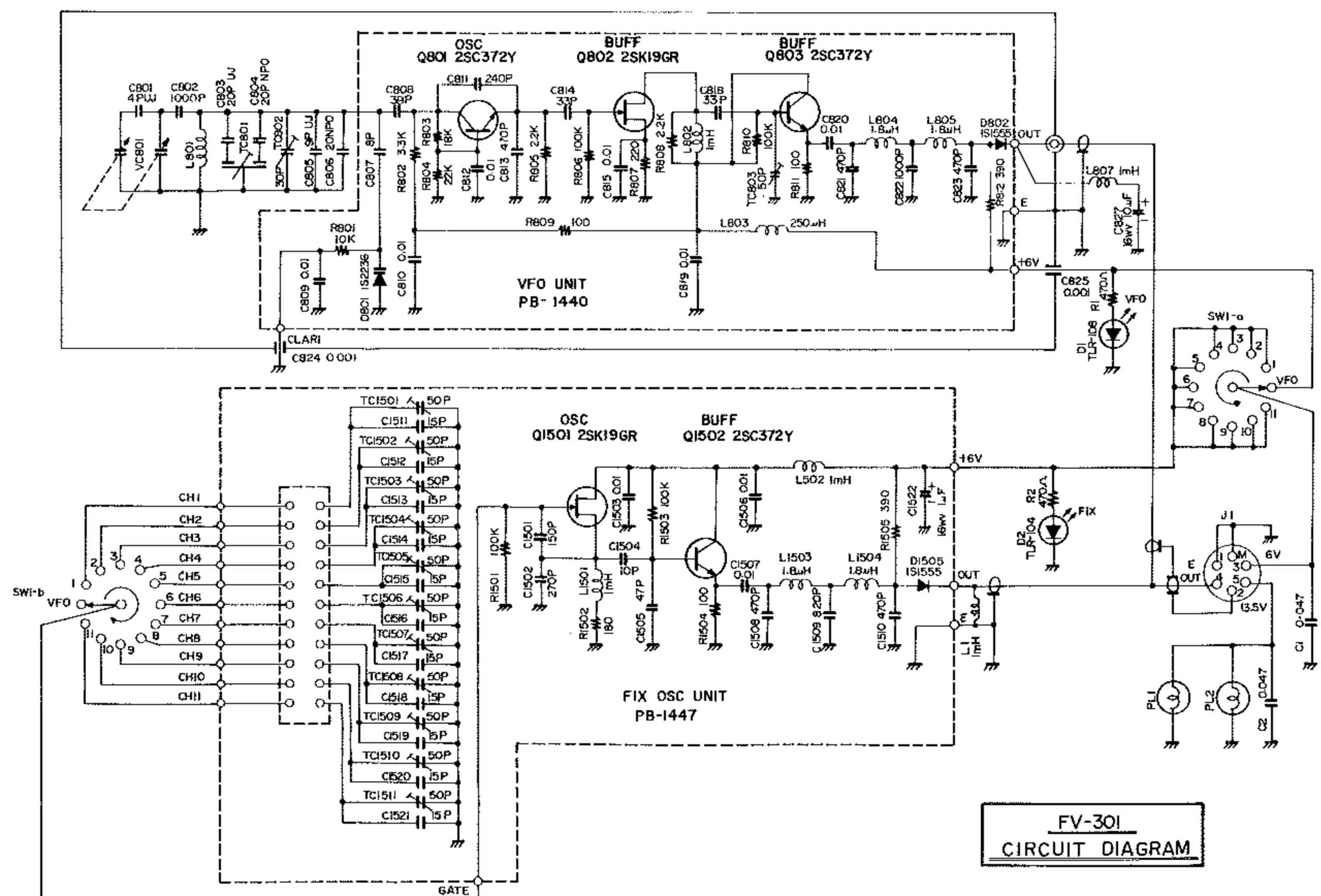
第32図 FV-301 回路図
