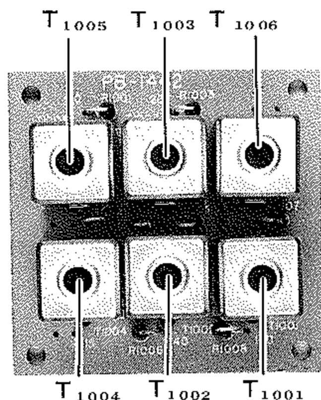
BPF UNIT (PB-1442)
