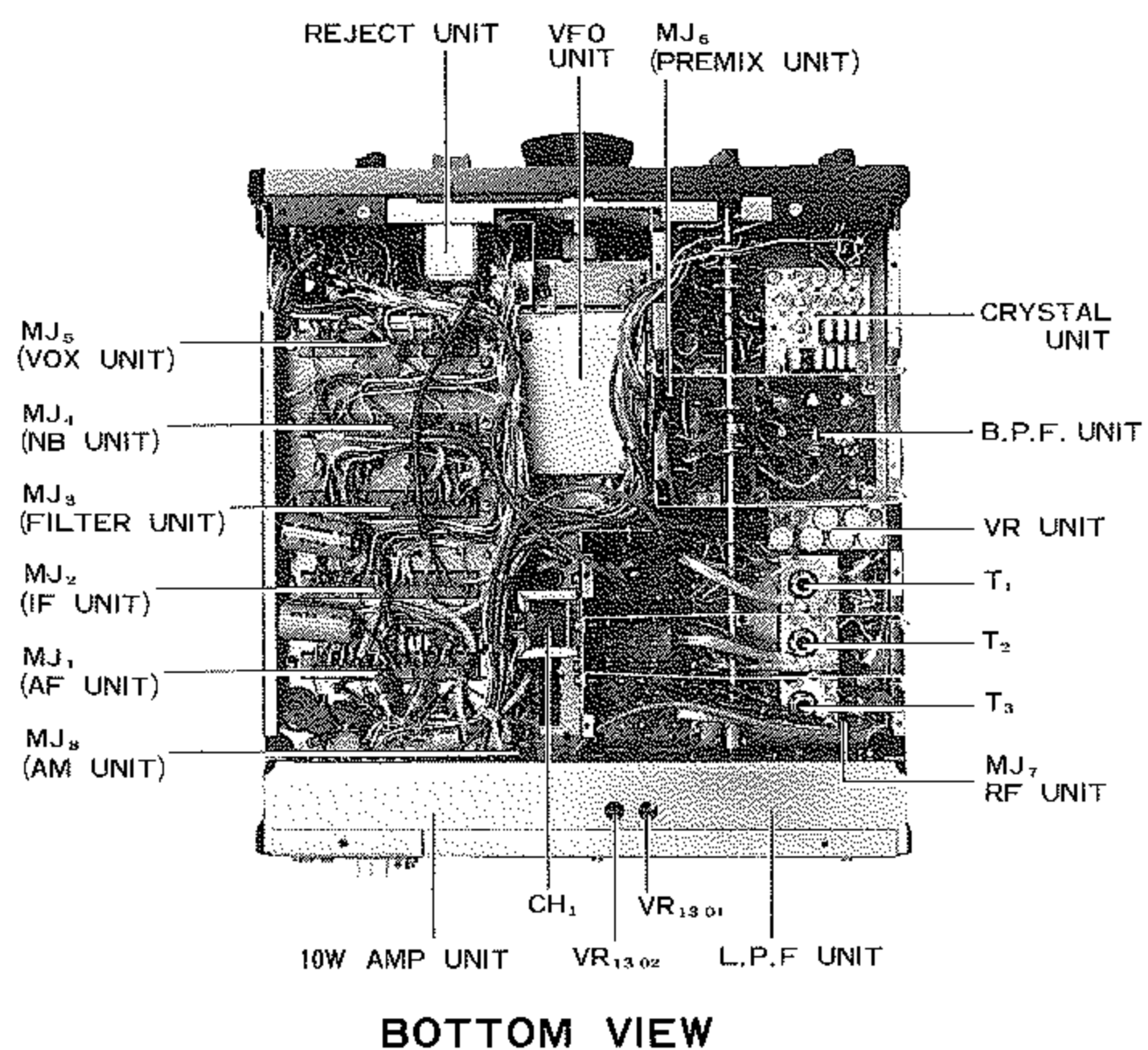
FT-301S 内部写真
