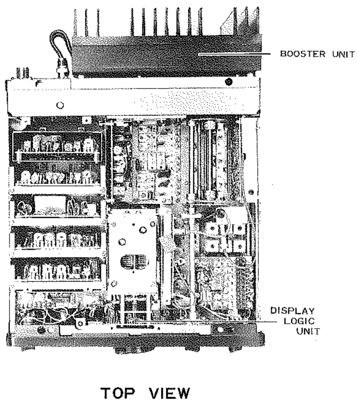
FT-301D 内部写真
