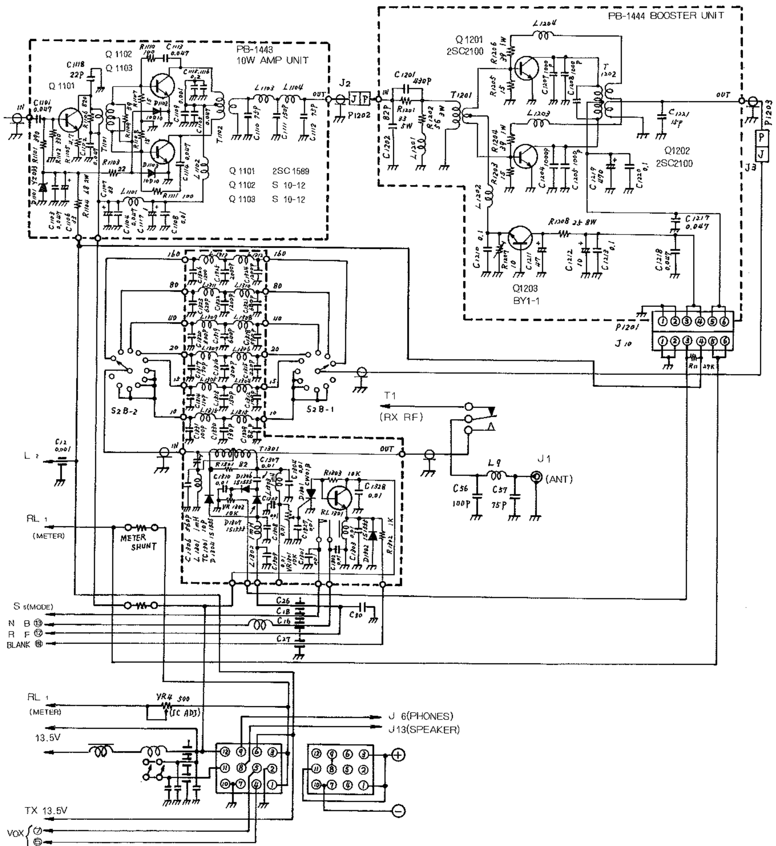
第30图 FT-301, FT-301D 終段部分
