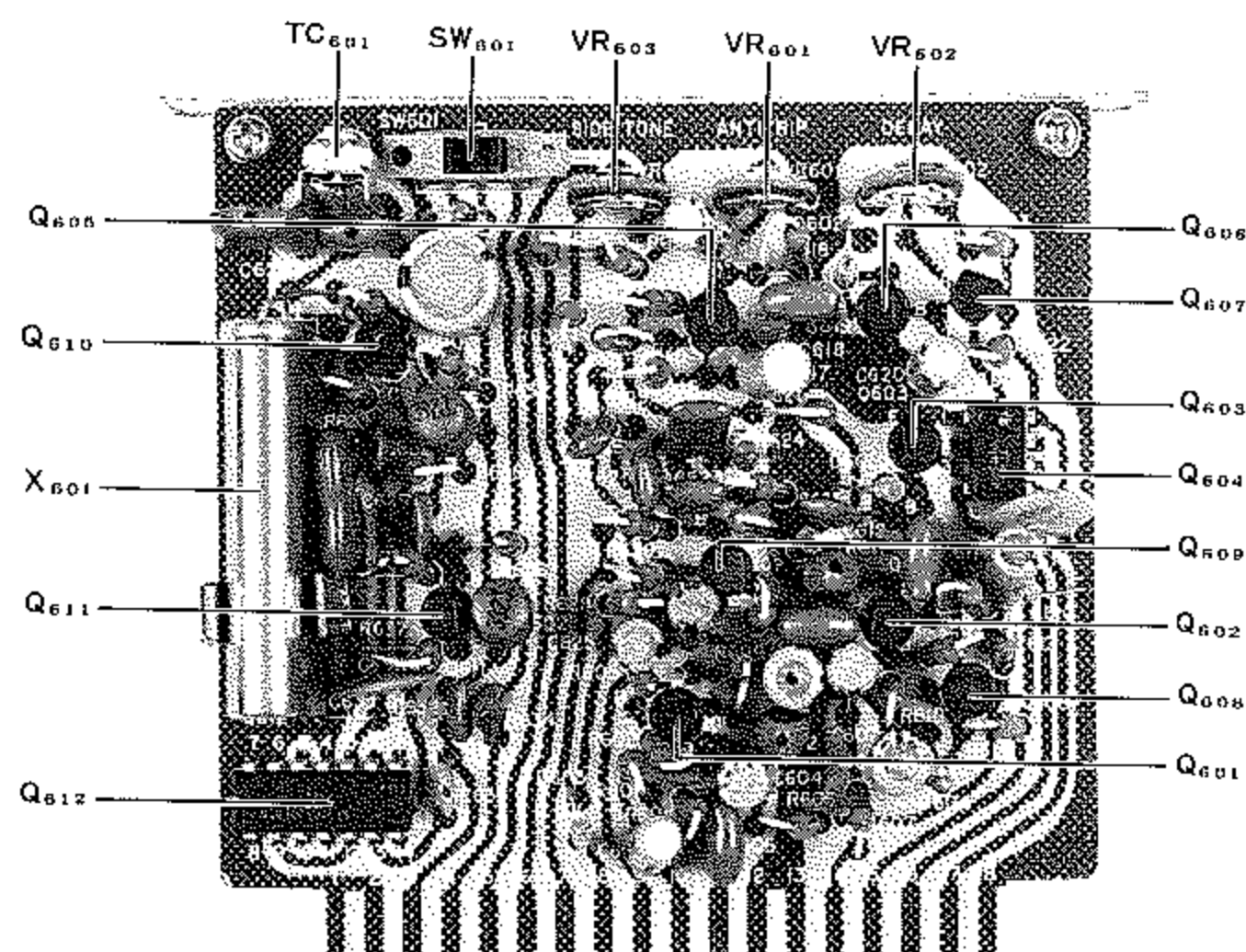
VOX UNIT (PB-1438)
