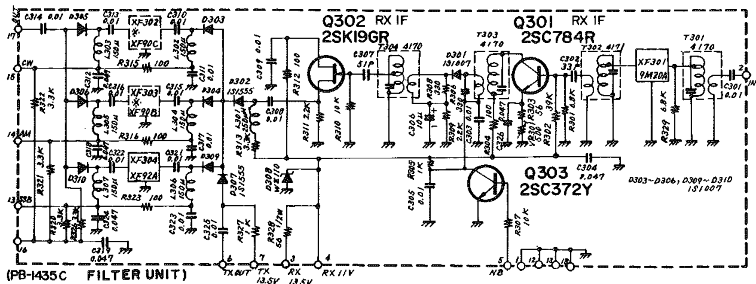
第11図 FILTER UNIT (PB-1435C)
