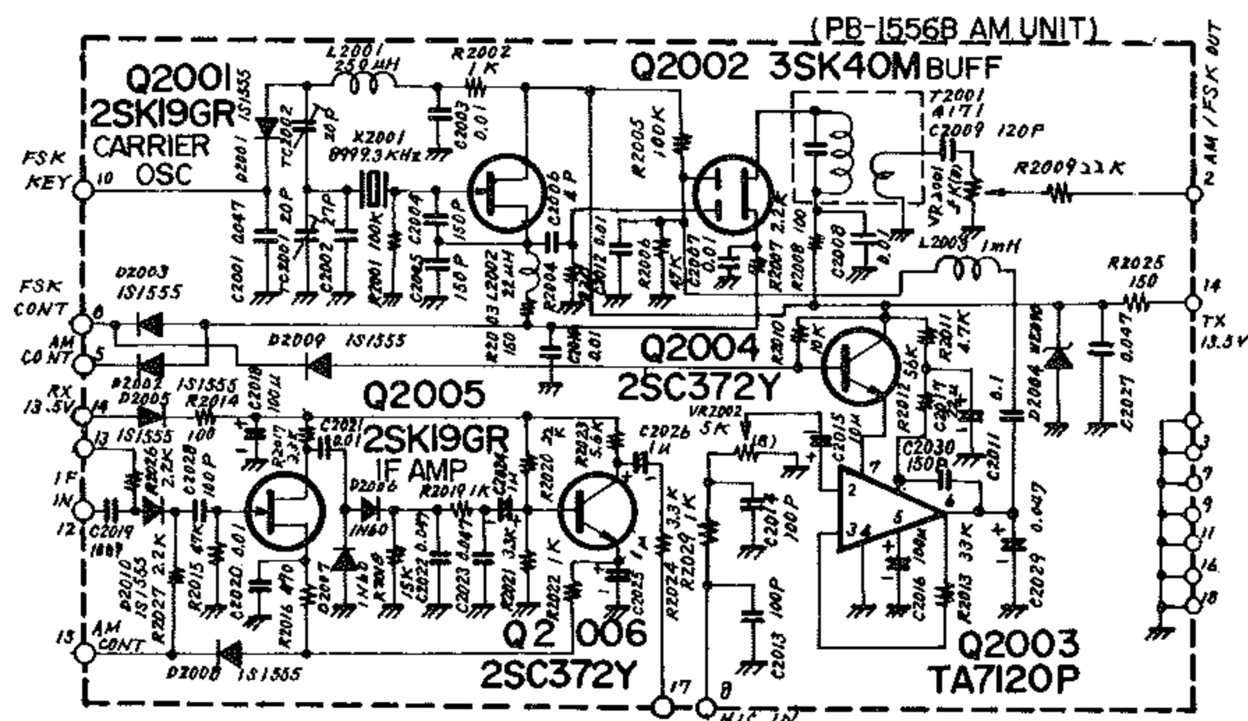
第14図 AM UNIT (PB-1556B)
