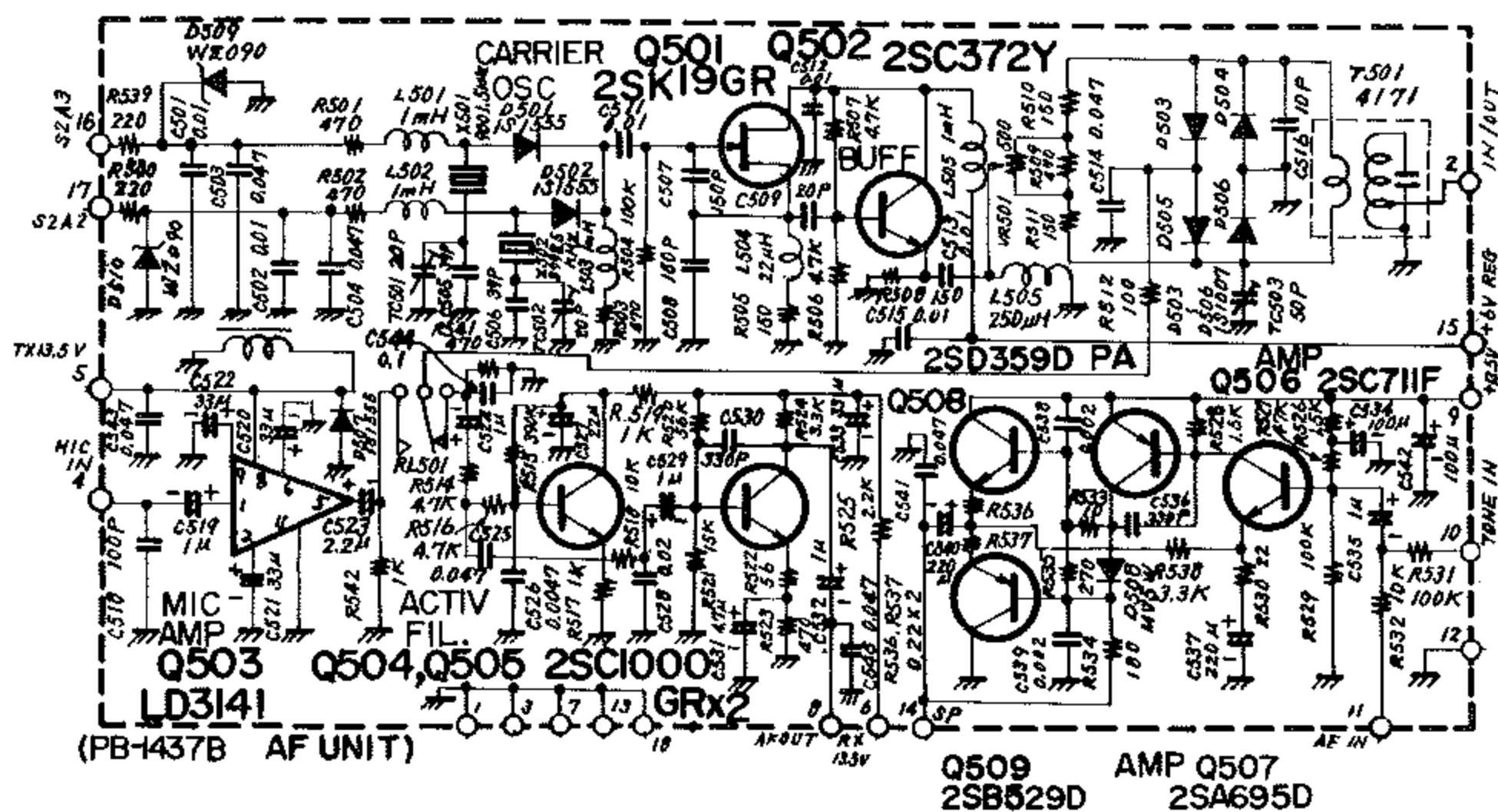
第13図 AF UNIT (PB-1437B)
