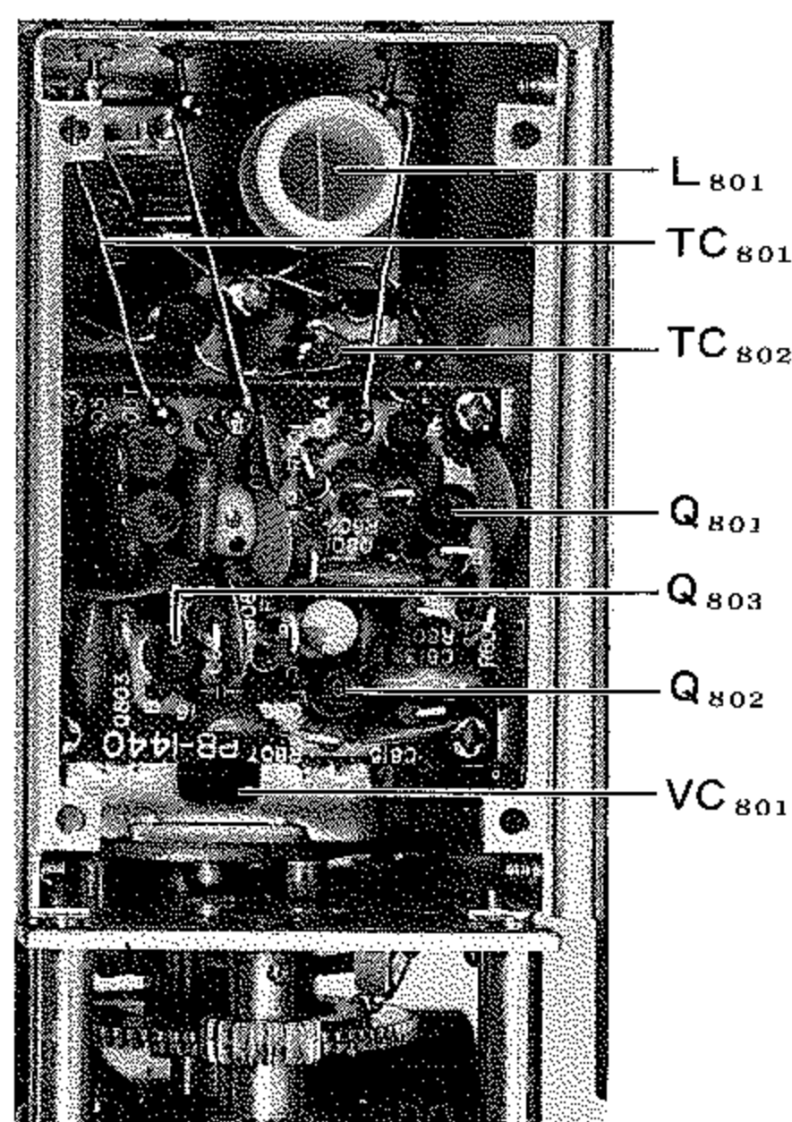
VFO UNIT
