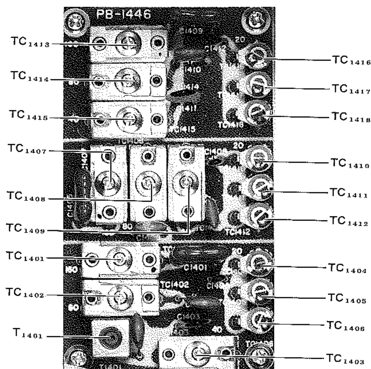
TRIMMER UNIT (PB-1446)
