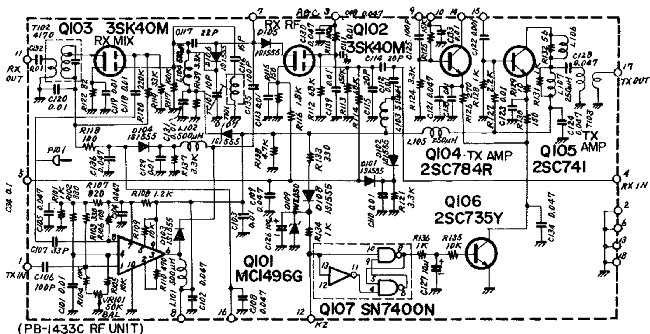
第10図 RF UNIT (PB-1433C)
