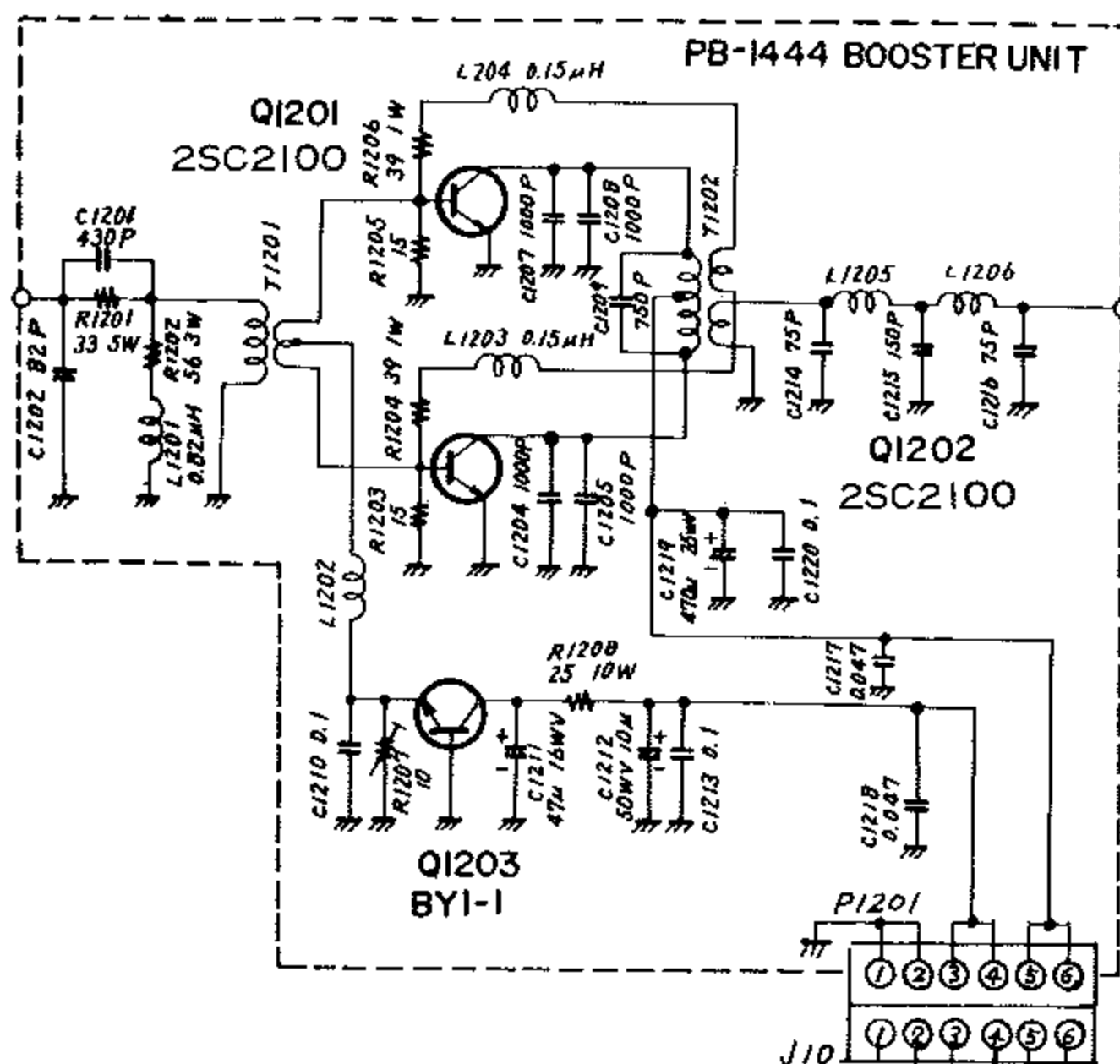
第18図 BOOSTER UNIT (PB-1444)
