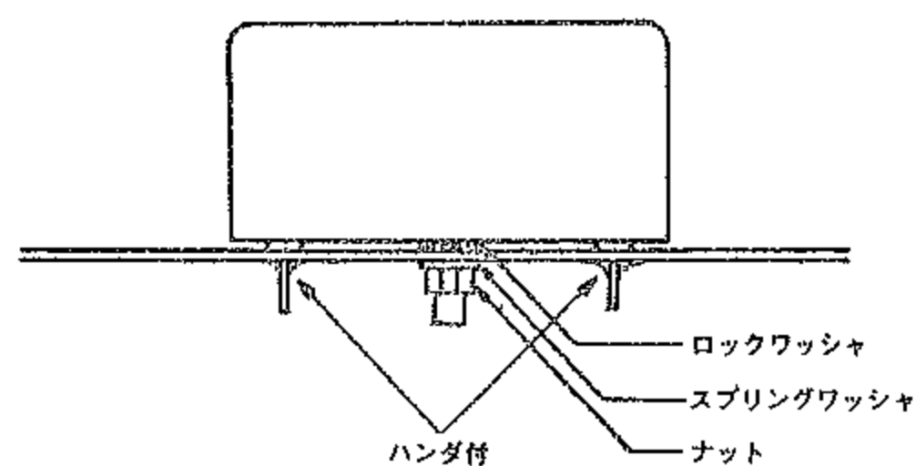
各フィルタの基板取付方法
