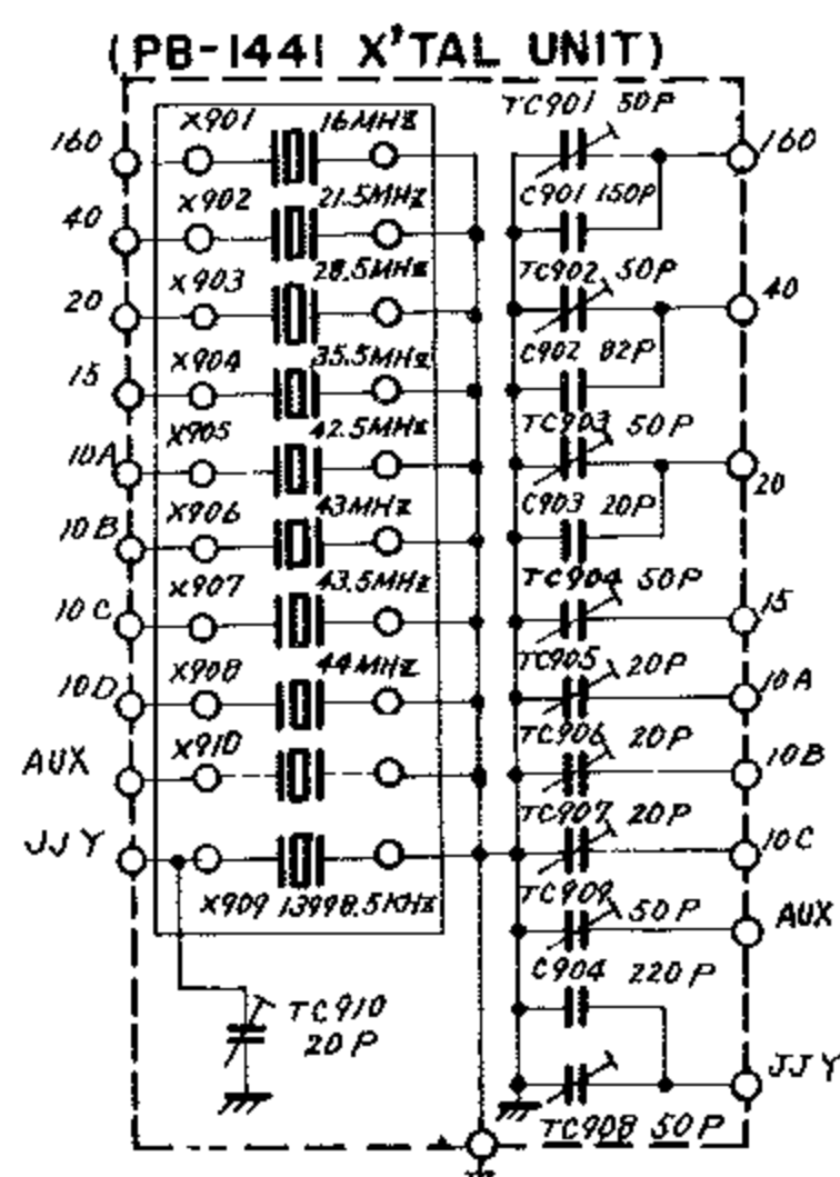
第25図 CRYSTAL UNIT (PB-1441)
