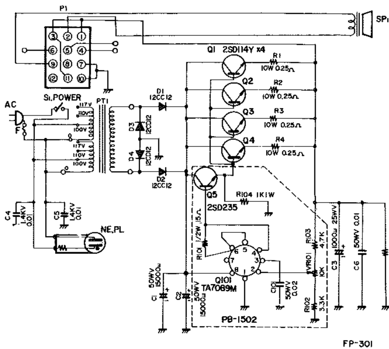
第33図 FP-301 回路図
