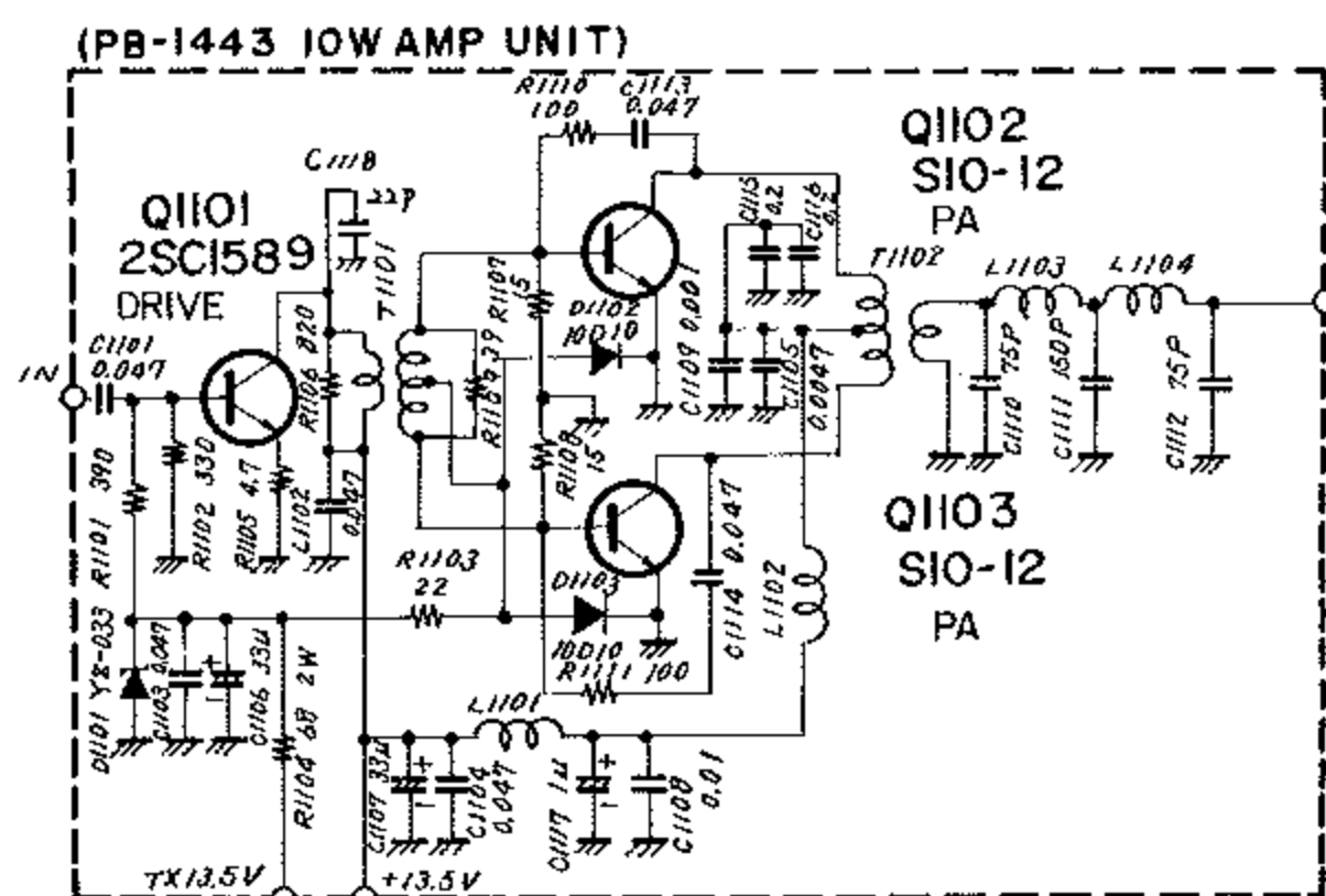
第16図 10W AMP UNIT (PB-1443)
