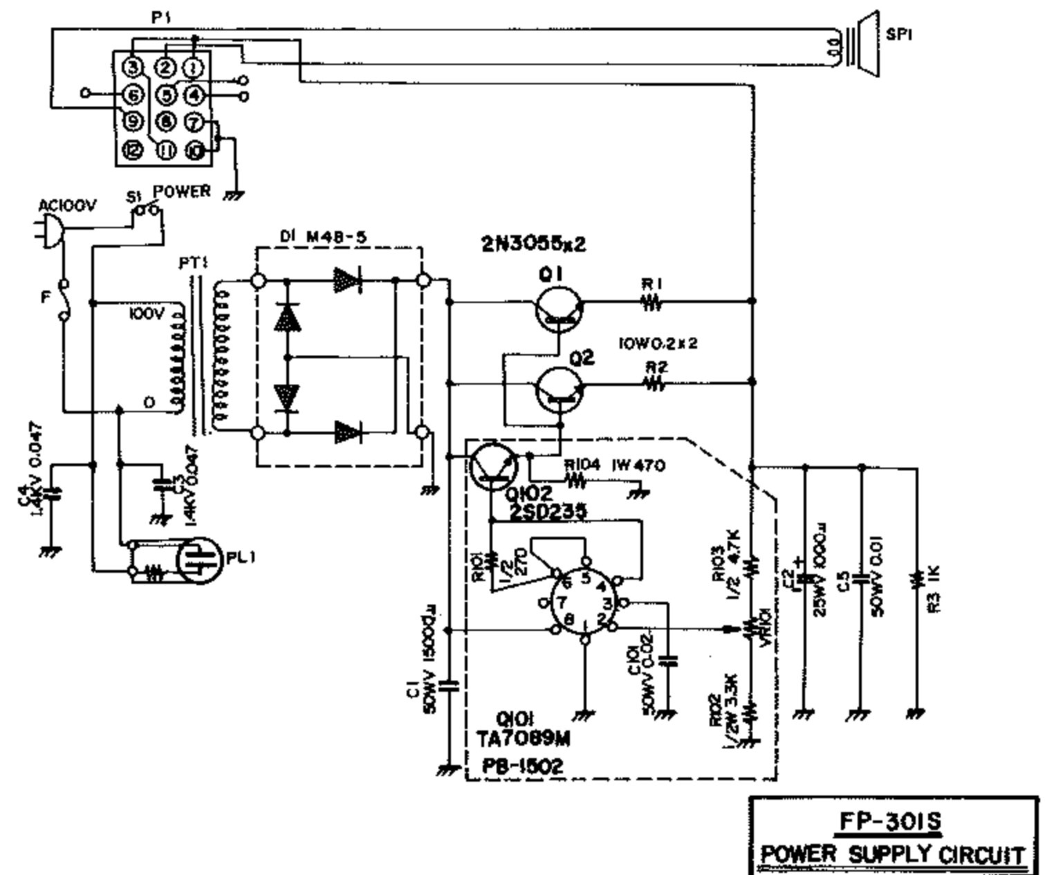
第34図 FP-301S 回路図
