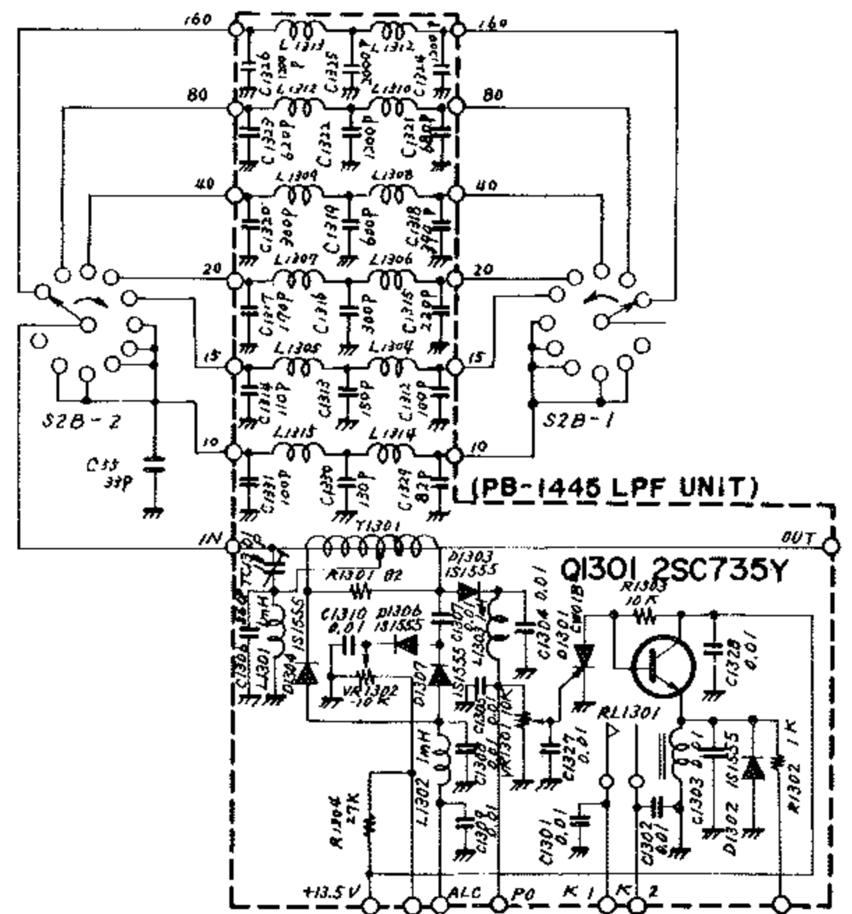
第19図 LPF UNIT (PB-1445A)
