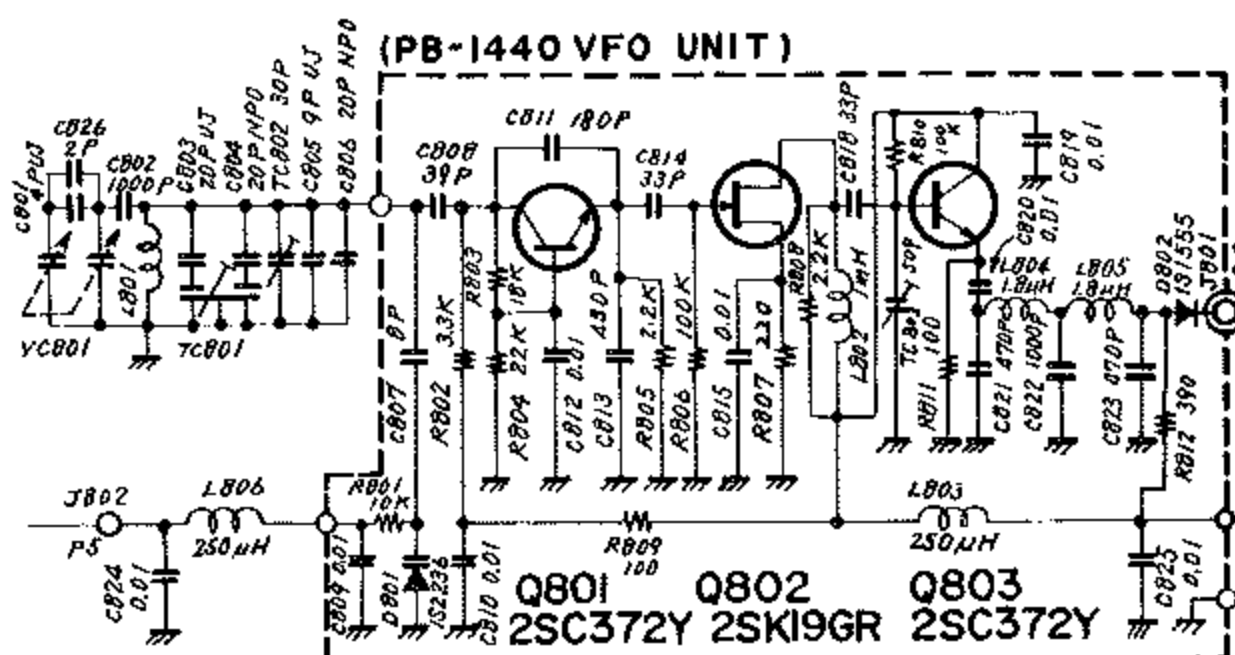
第22図 VFO UNIT
