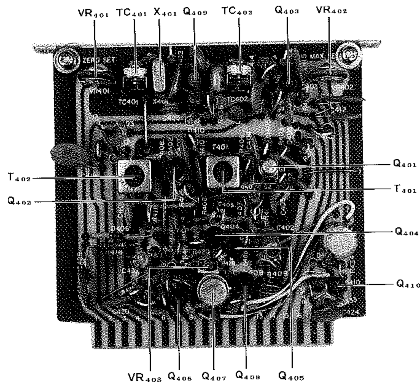
IF UNIT (PB-1436)
