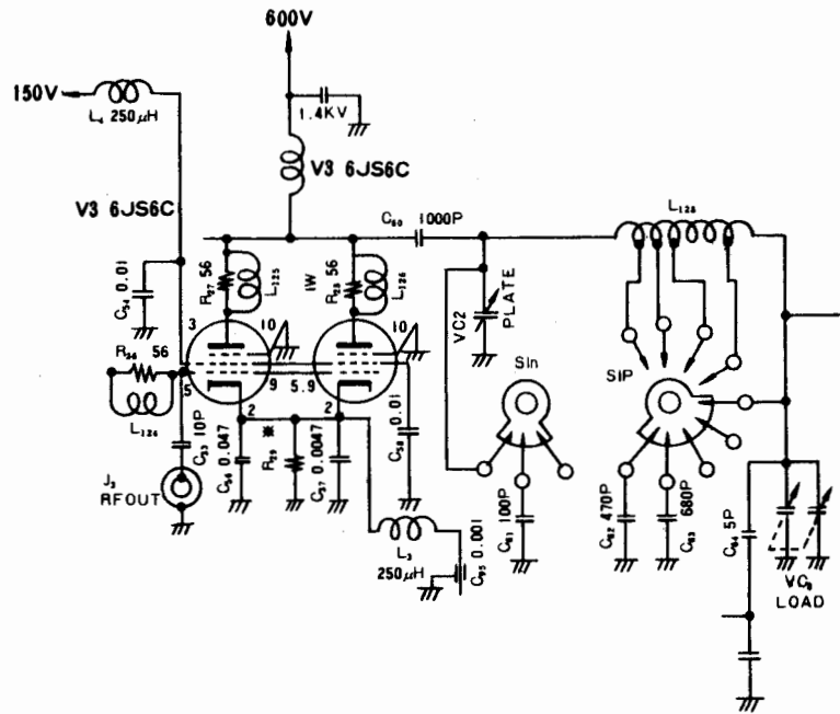
第13図(A)
