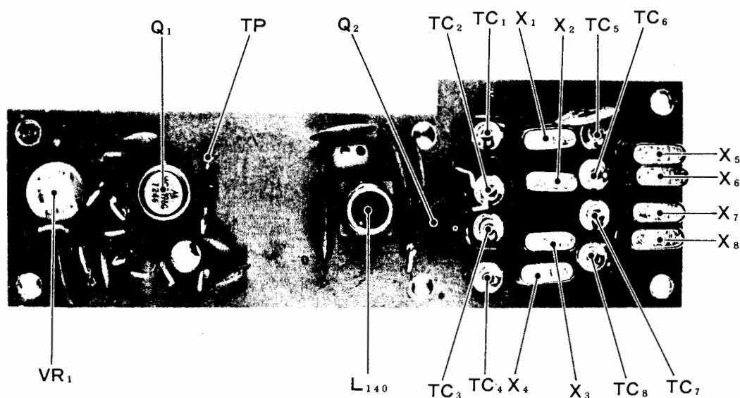
PREMIX UNIT(PB-1383)
