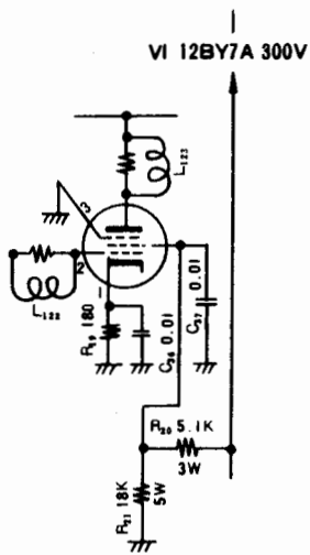
第12図(A)
