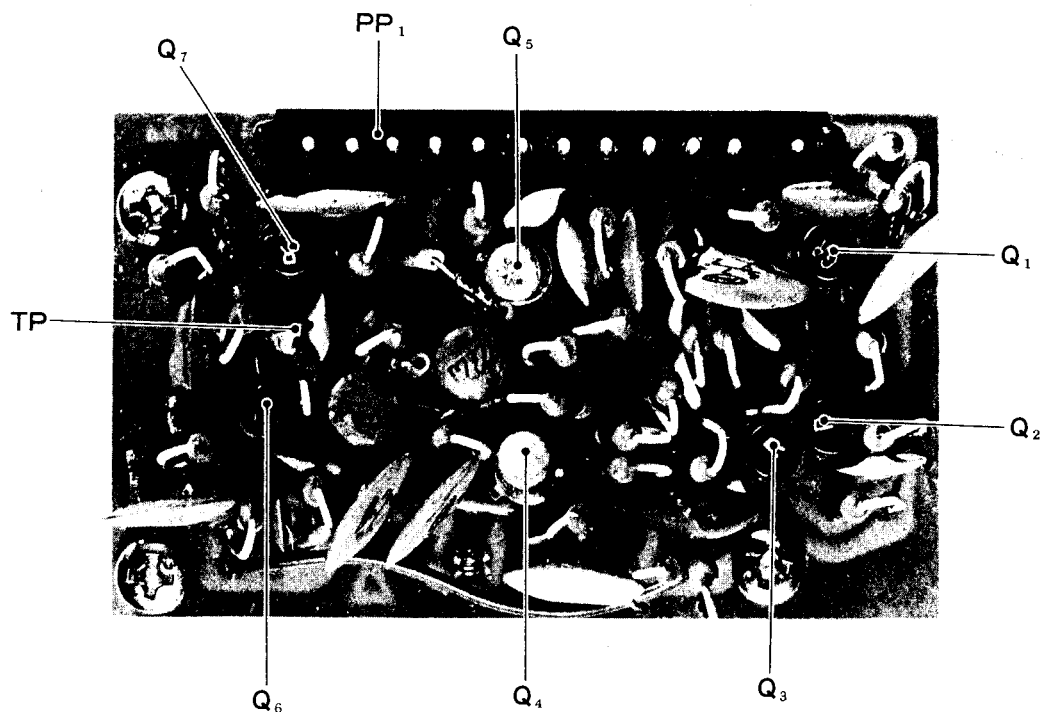
RF UNIT(PB-1381)
