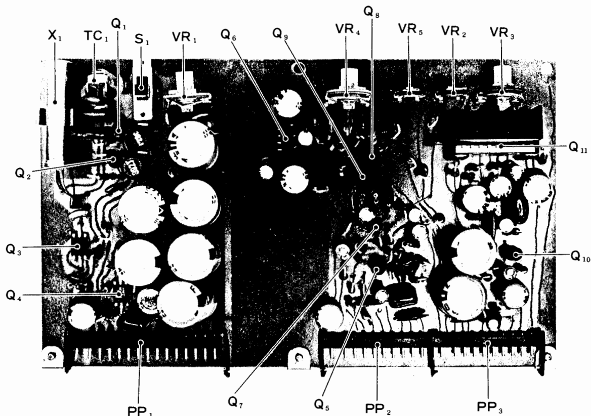
AF UNIT(PB-1385)
