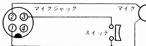
第2図 マイクの接続
