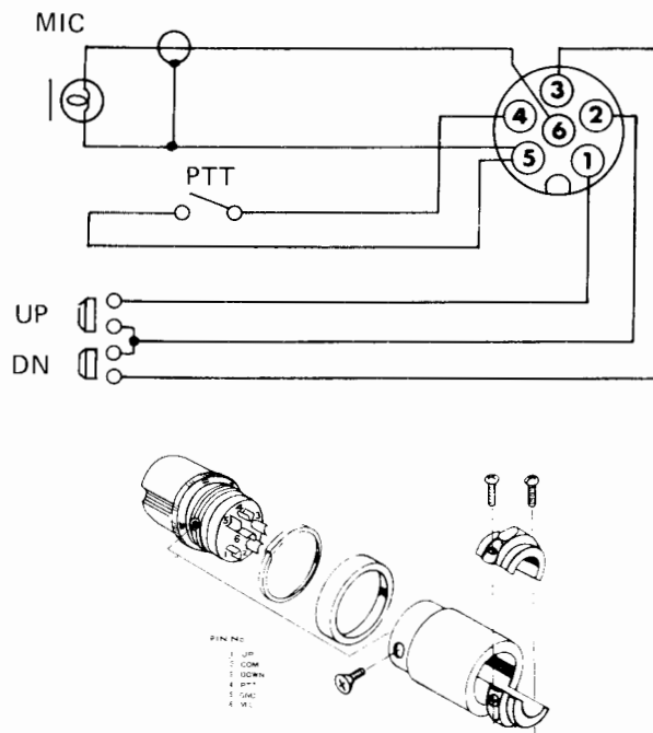
第1図 スキャニングマイクロホンの接続
