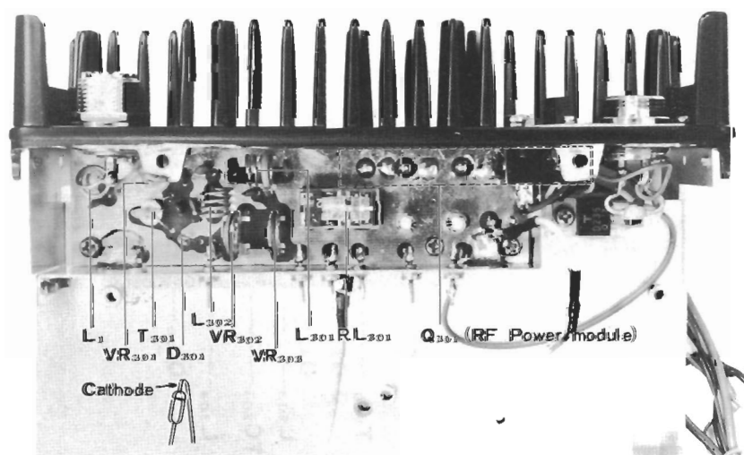
BOOSTER UNIT(PB-1793)
