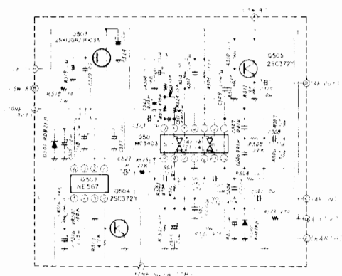
第7図 Tone Squelch 回路図
