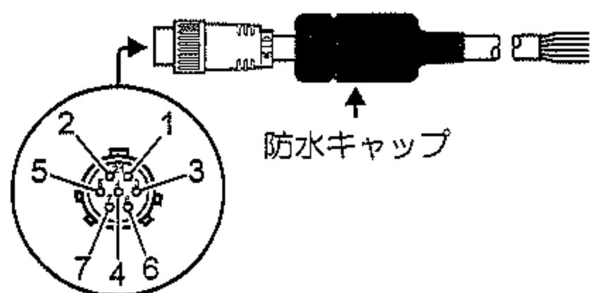
7Pメタルコネクタの端子番号
