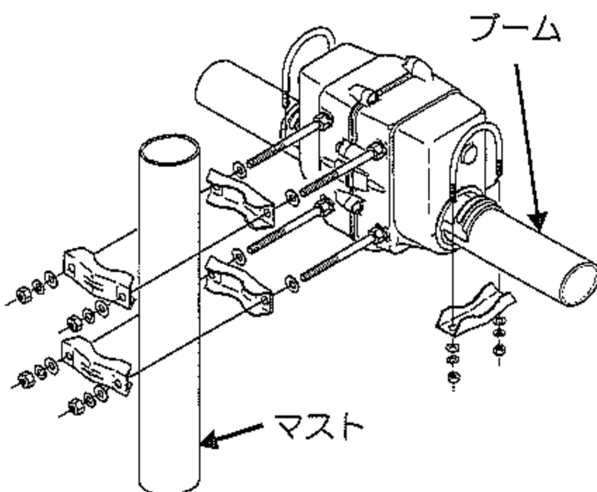
取付例
