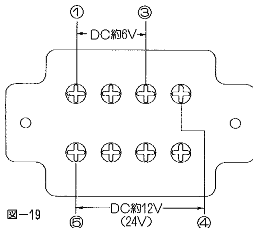
G-450コントローラー側ケーブルコネクタ
