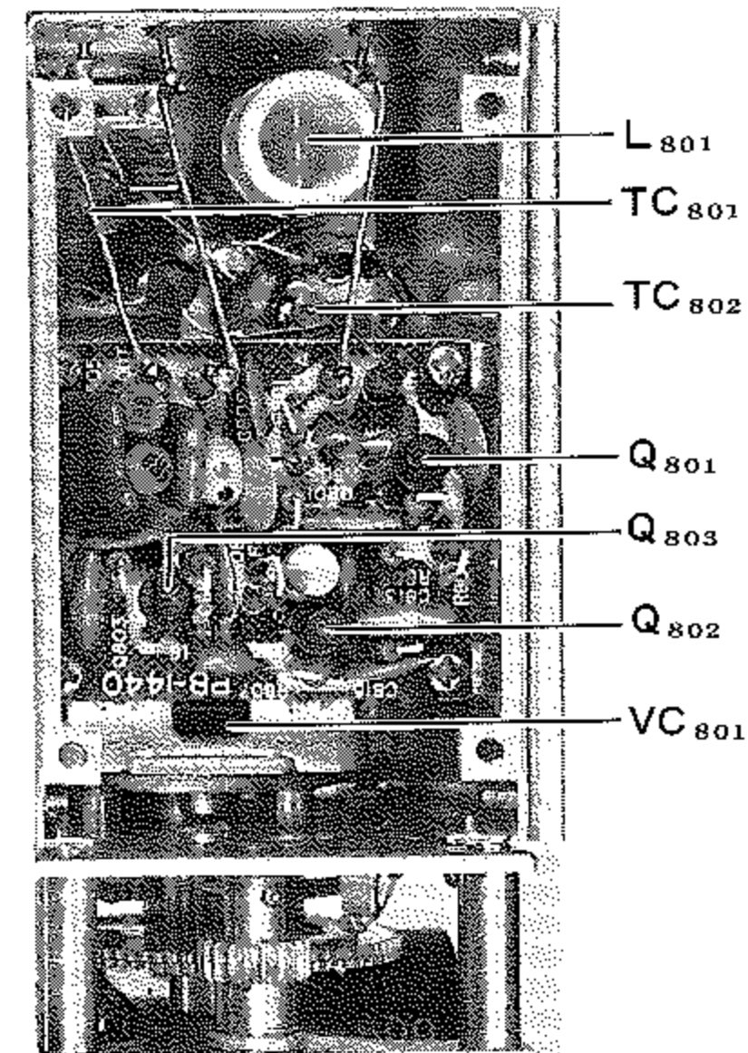
VFO UNIT
