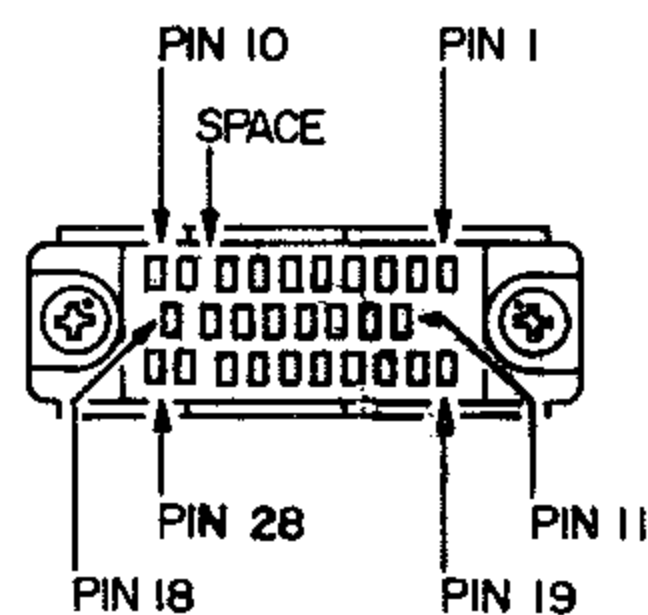
(ACC-1 ソケットピン番号)
