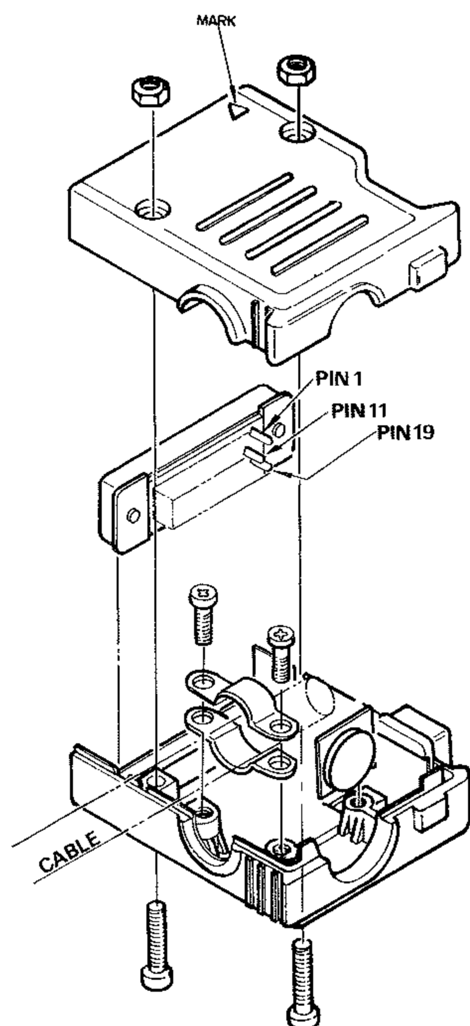
ACC-1 プラグの接続
