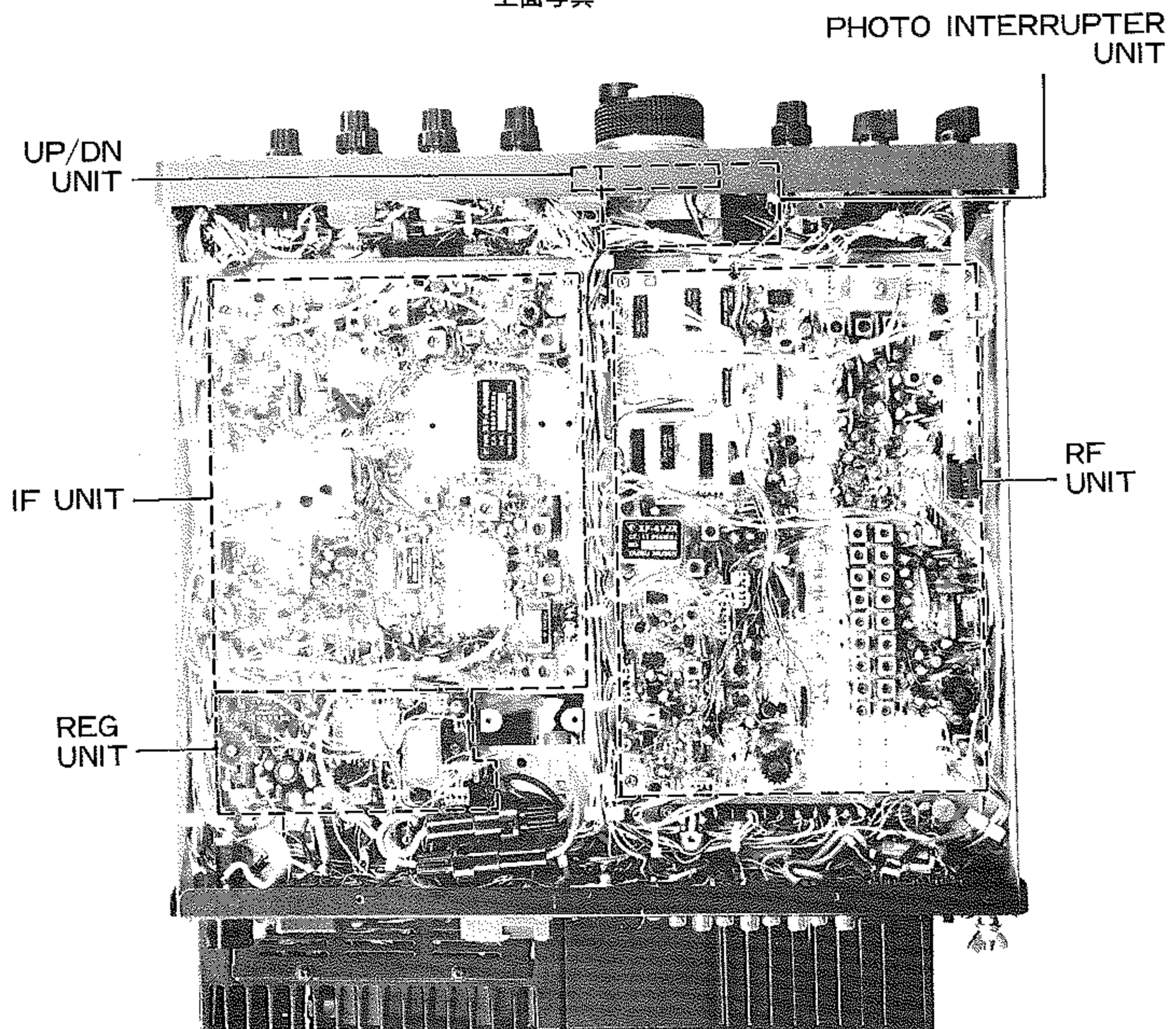
底面写真
