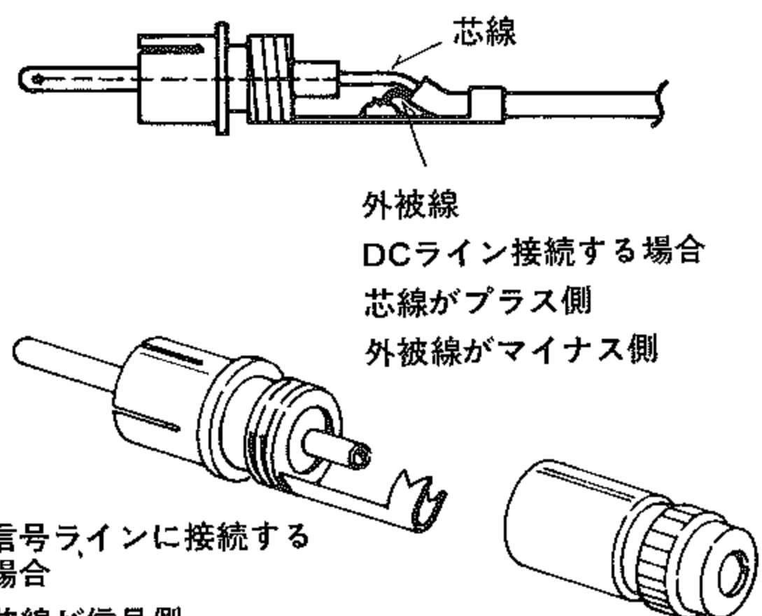
ピンプラグの接続
