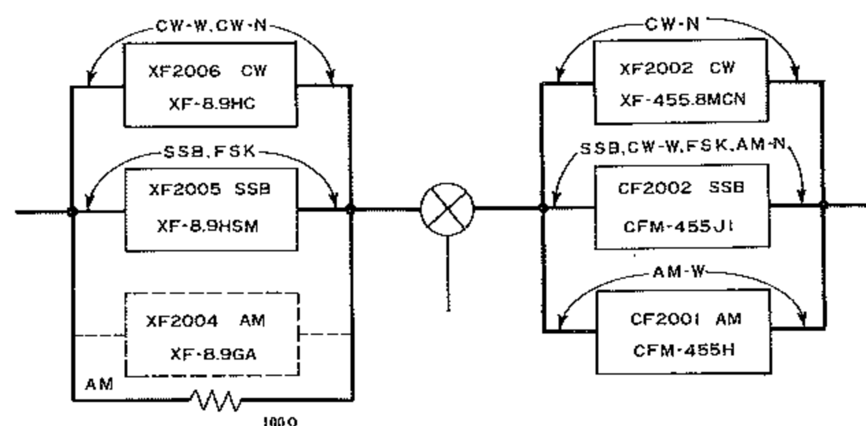
④ CW-W, XF-8.9HCおよび CW-N, XF-455.8MCN実装時
