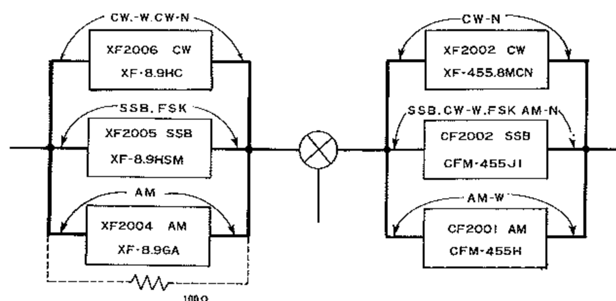
⑥ 全フィルタ実装時
