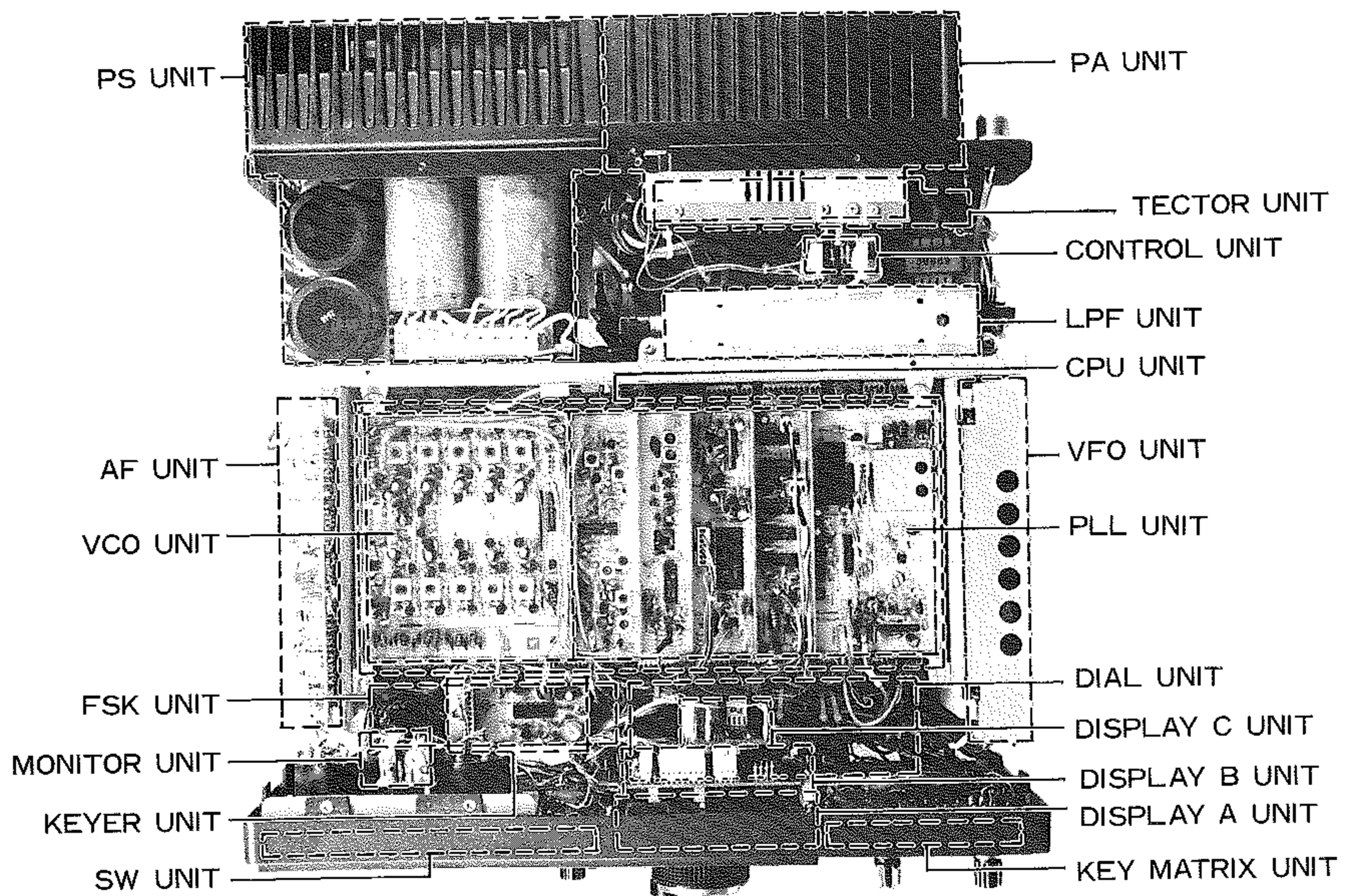
上面写真
