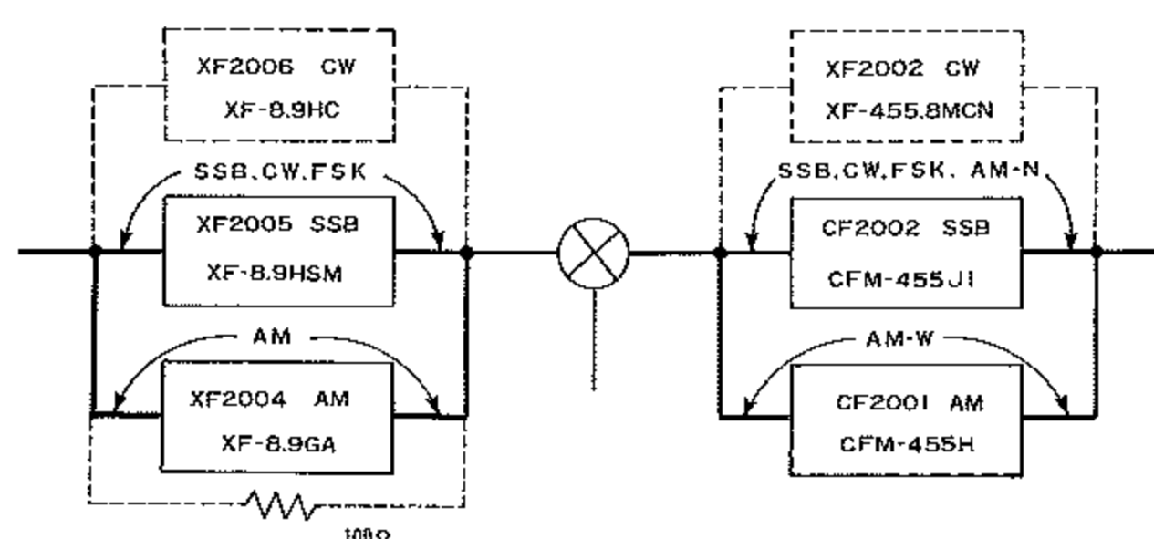
⑤ AM-W, XF-8.9GA実装時
