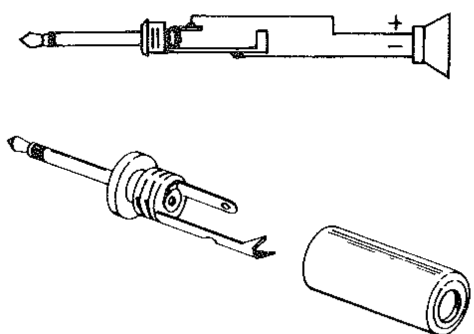
外部スピーカプラグの接続
