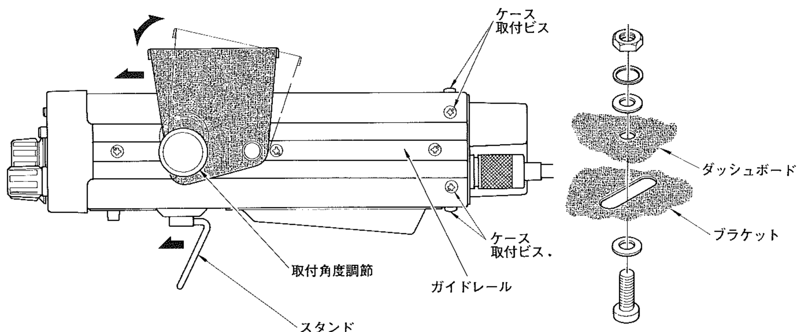
第4図 マウントブラケットの取り付け方
