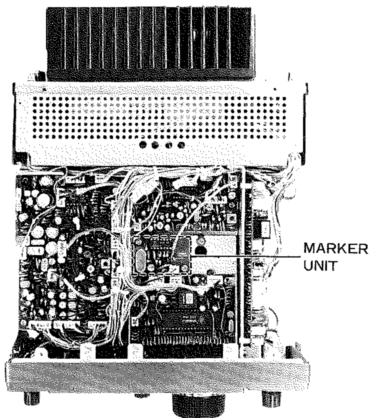
上面側
