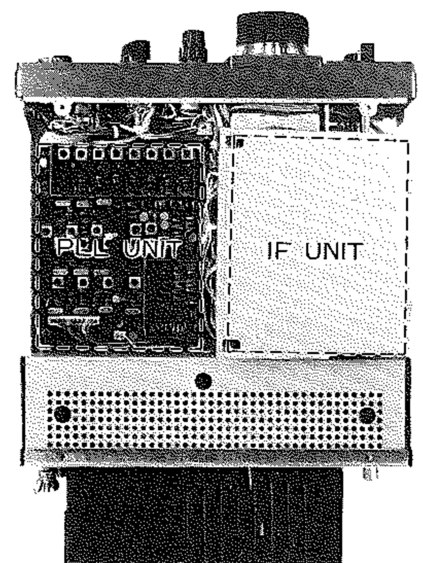
底面側IFユニットを外した状態
