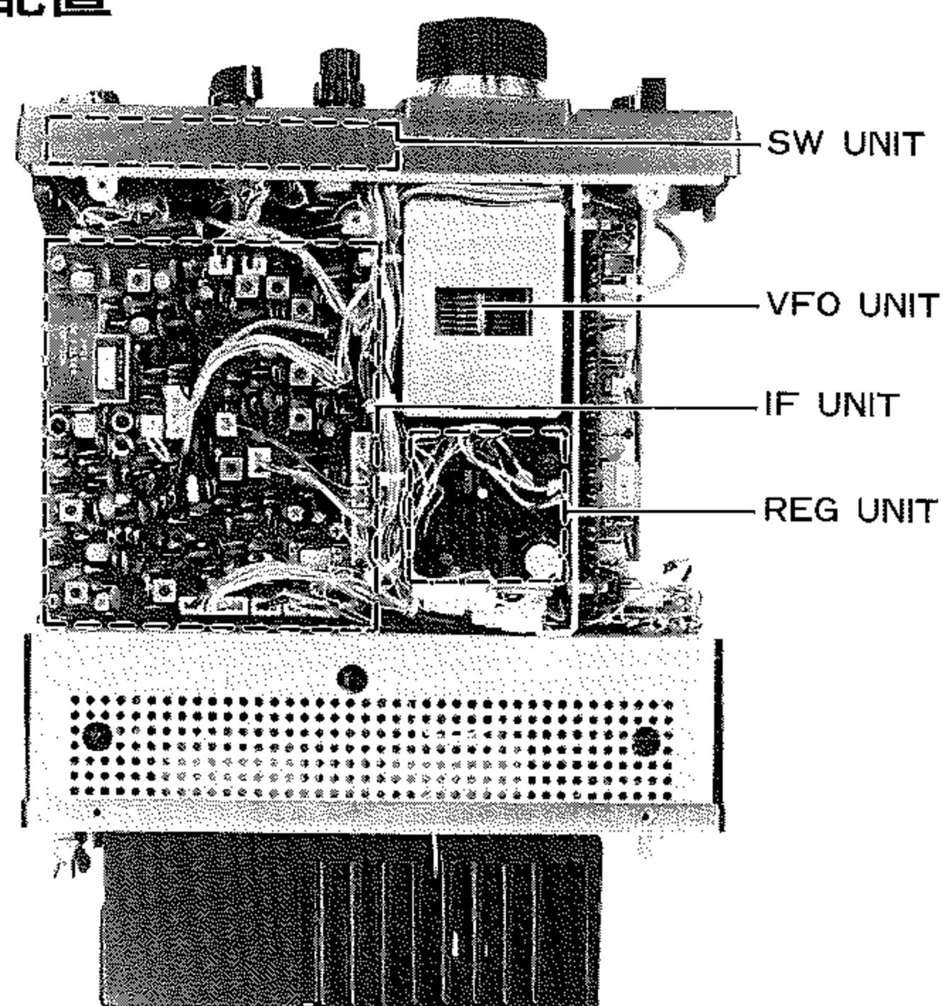
底面写真
