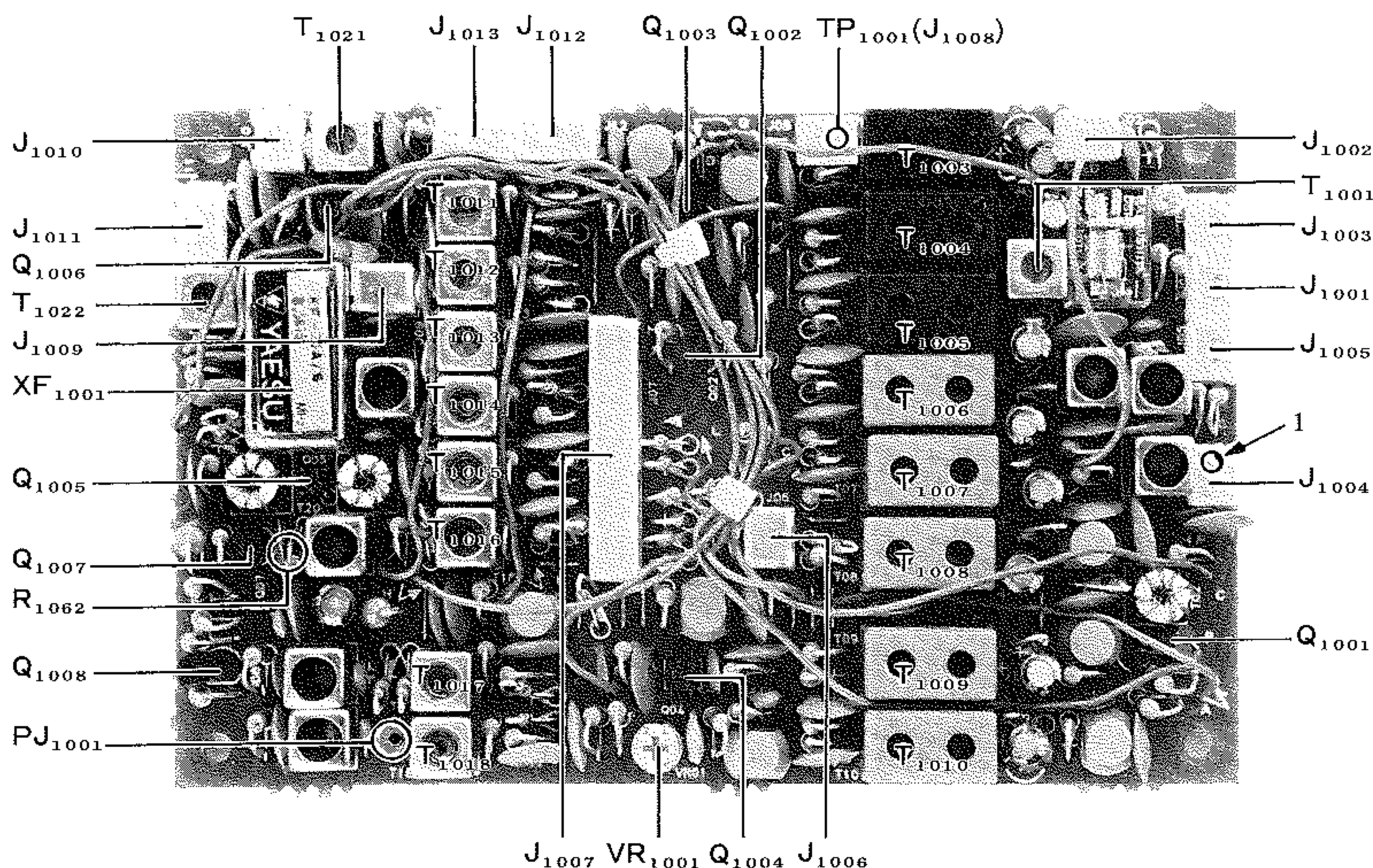
RF ユニット
