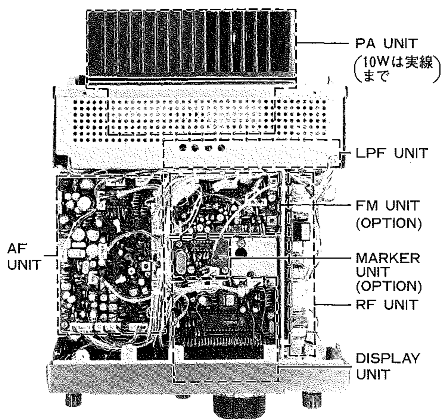
上面写真
