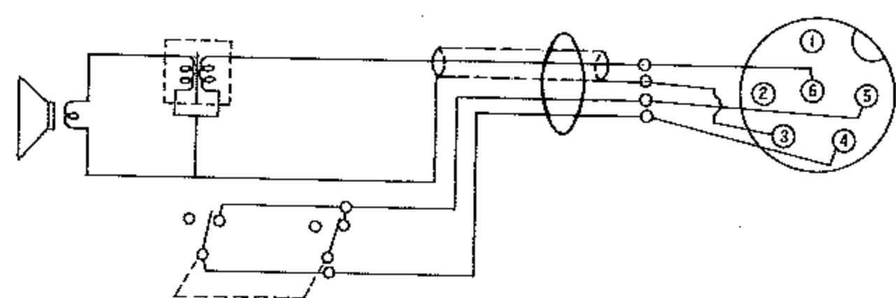
第 3 図 マイクの接続
