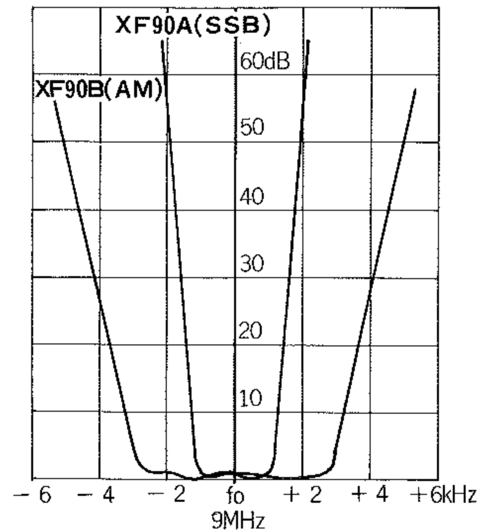
第6図 水晶フィルタの特性
