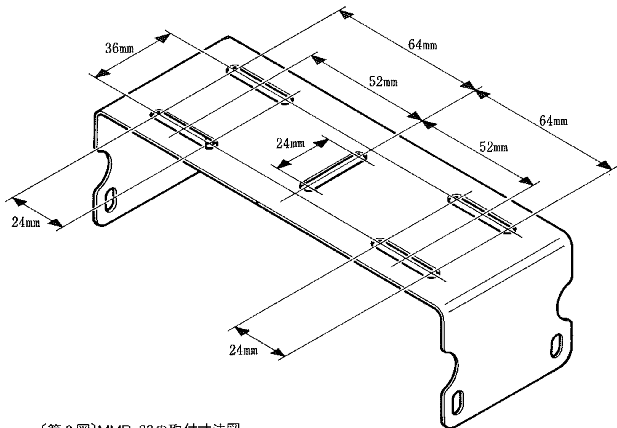
〔第2図〕MMB-33の取付寸法図
