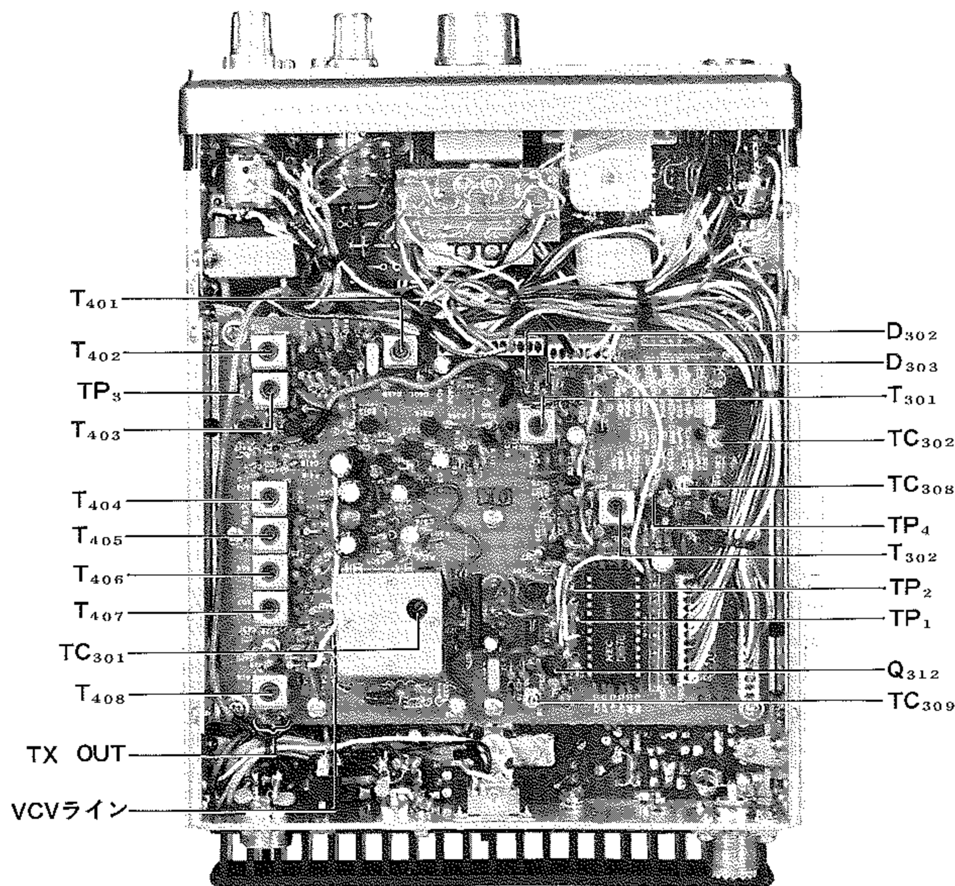
PLL 部調整箇所
