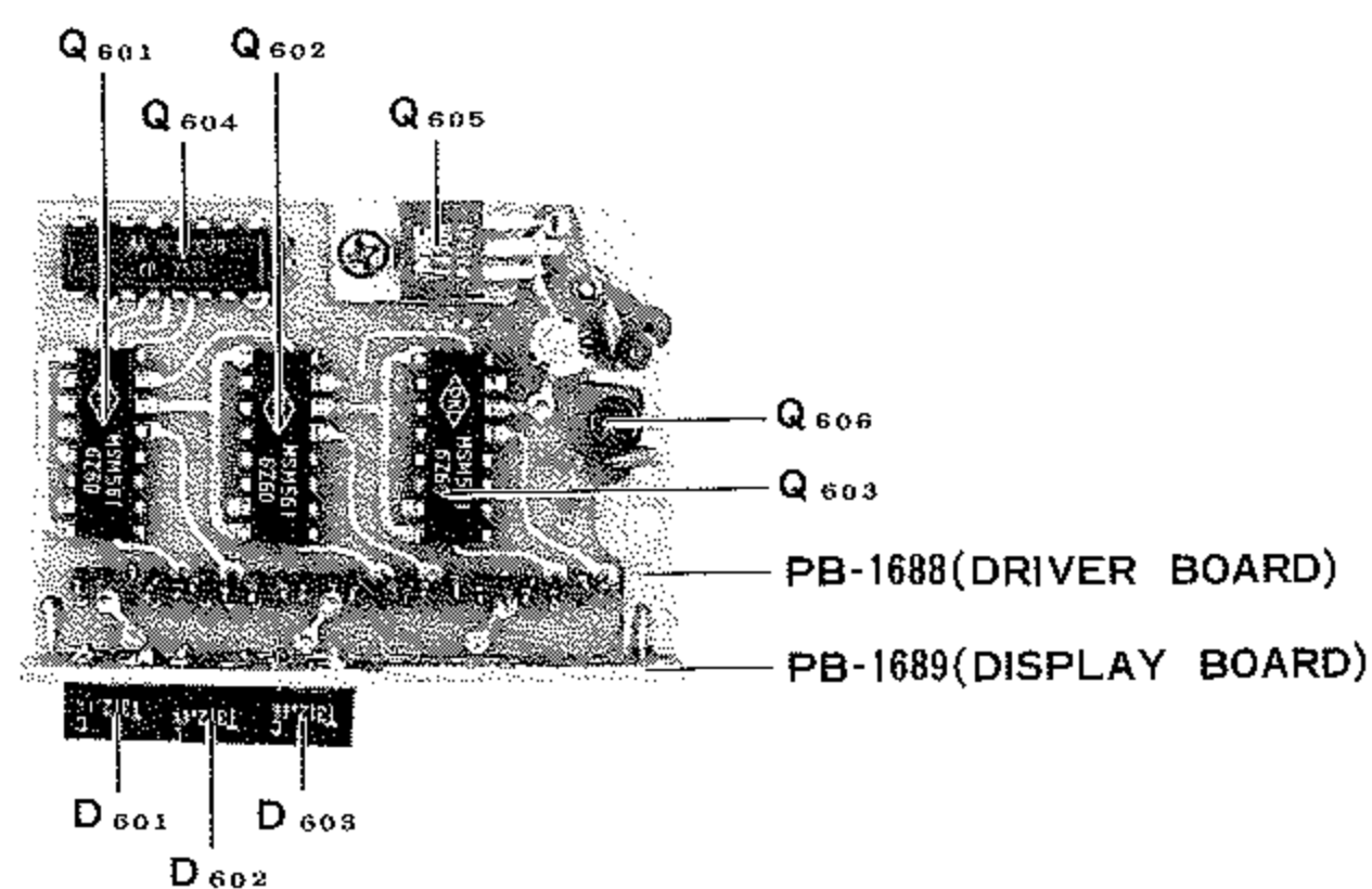
DISPLAY UNIT (PB-1688, 1689)
