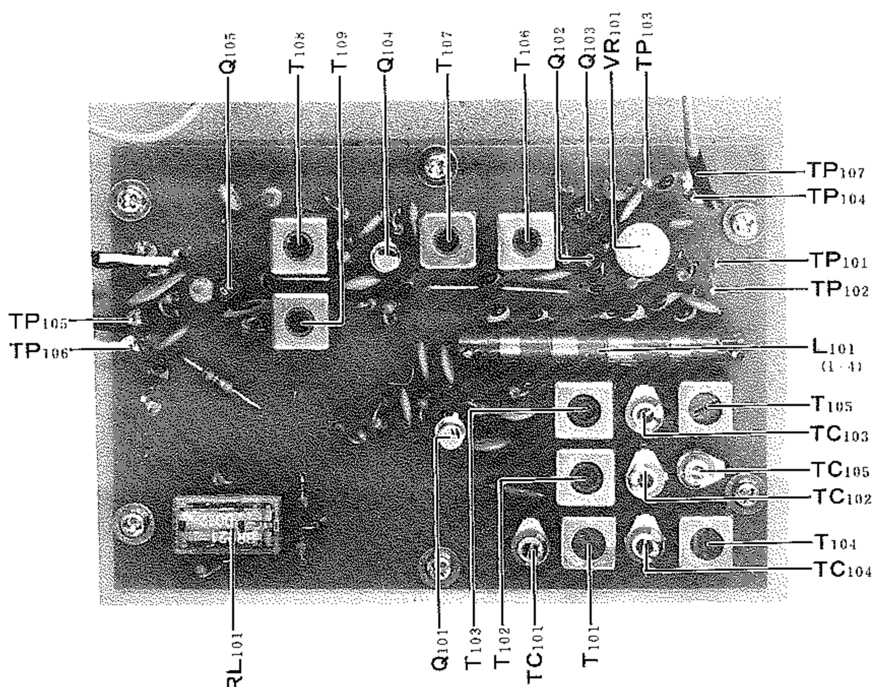
RF UNIT(PB-1781)
