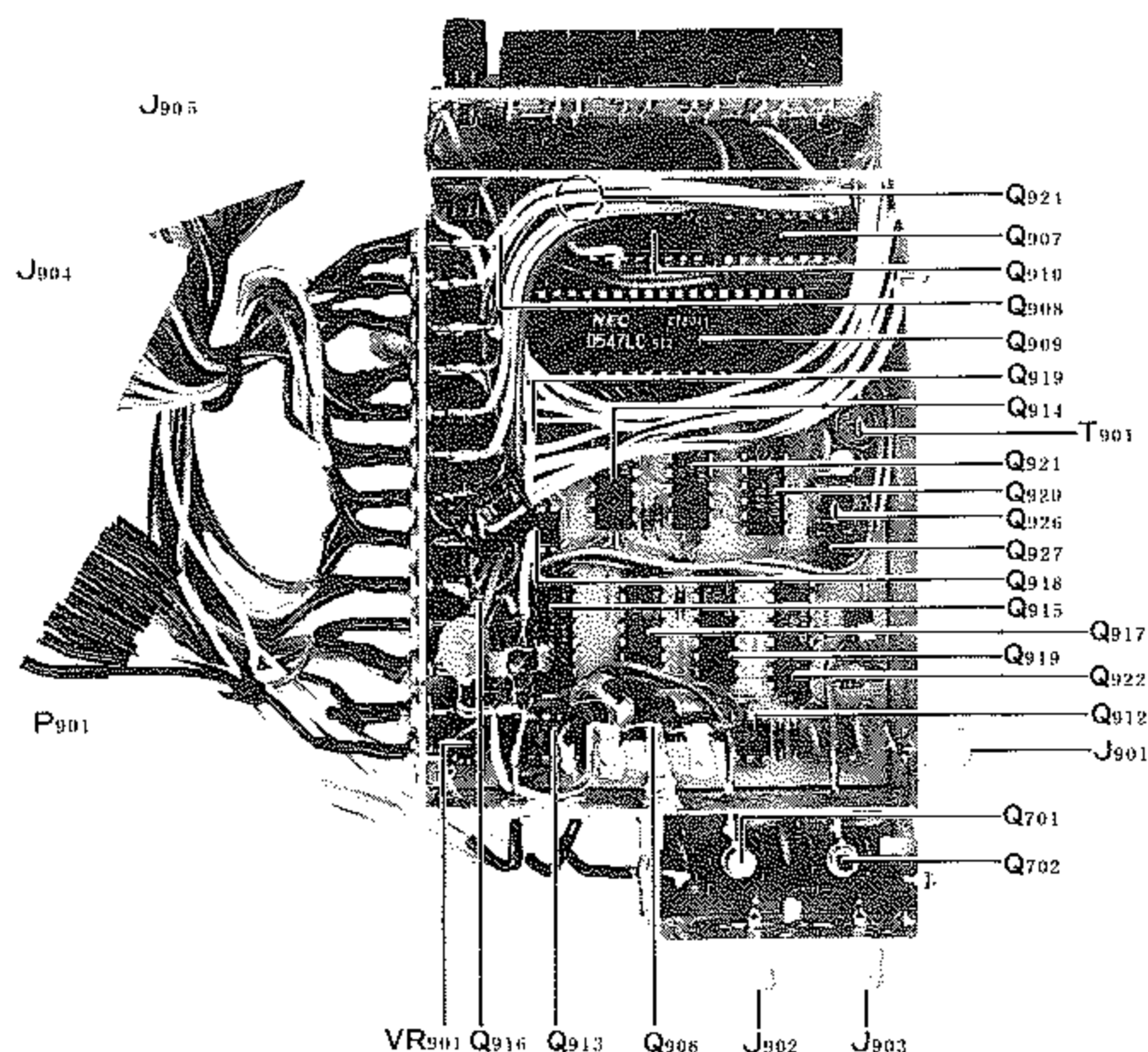
COUNTER UNIT (PB-1754)
