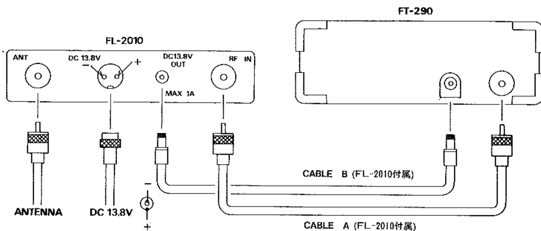
FL-2010/FT-290の接続
