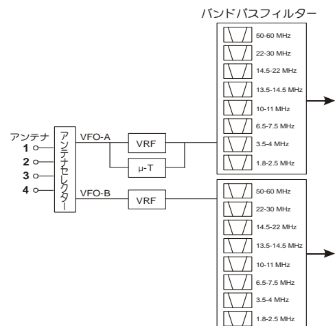
μ-TUNE/VRF回路 概念図
