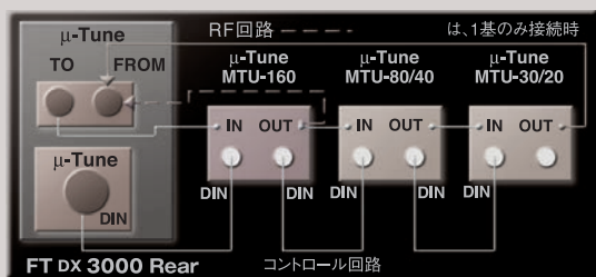
RFμチューニングキット接続図
