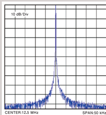
C/N比特性
