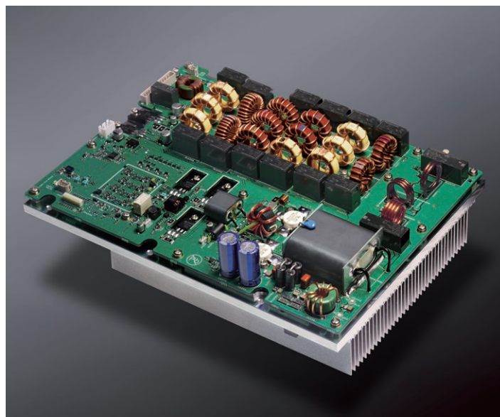
200W PAユニット
