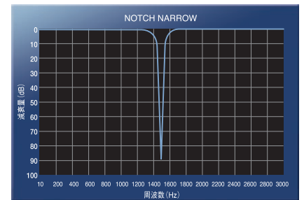
IF NOTCH特性
