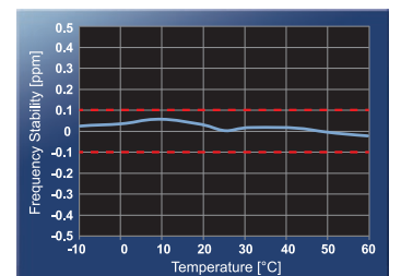
TCXO 温度特性
