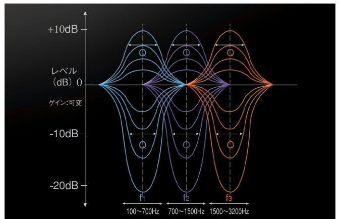
パラメトリックイコライザー概念図
