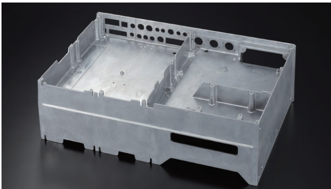
大型アルミダイキャストシャーシ
