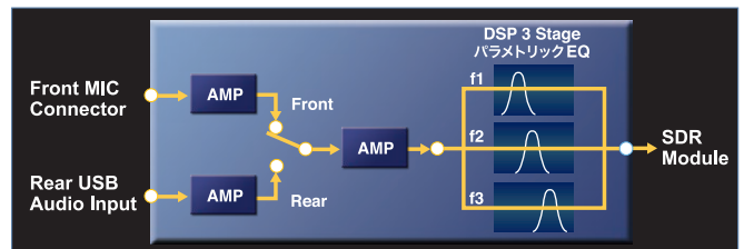
マイク回路ブロックダイヤグラム
