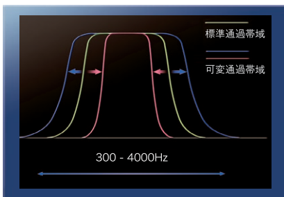
IF WIDTH 動作概念図 (USB/LSB)
