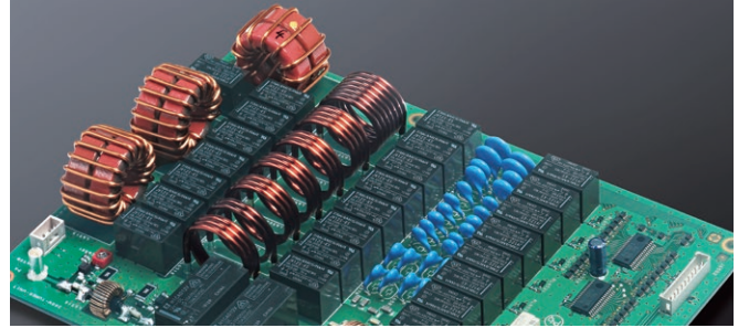
高速オートマッチングアンテナチューナー (写真はMPバージョン)
