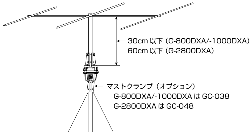
14MHz 3 エレ八木アンテナの場合
