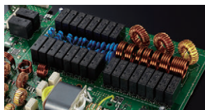
オートマチックアンテナチューナー
