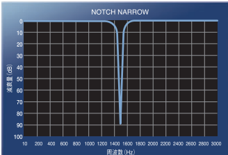
IF NOTCH 特性
