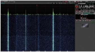
バンドスコープ(ウォーターフォール)表示
