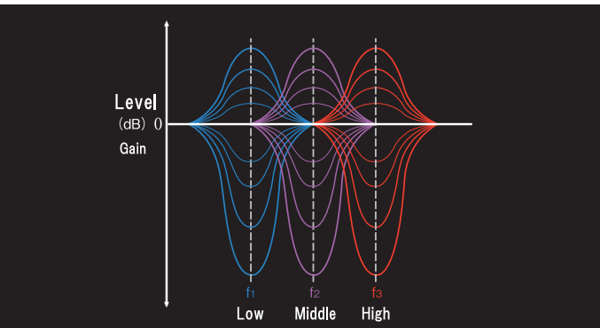
受信オーディオ パラメトリックイコライザー概念図
