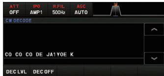
CWデコード表示
