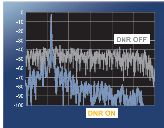
DNR (デジタルノイズリダクション) 特性
