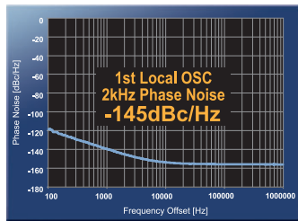
1st Local OSC フェーズノイズ (14.2MHz)
