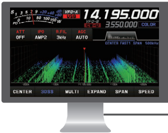
バンドスコープ(ウォーターフォール)表示
